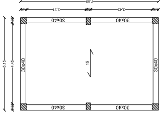
Impalcati 5° livello-Castelletto
