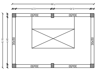
Impalcati 4° livello-Castelletto
