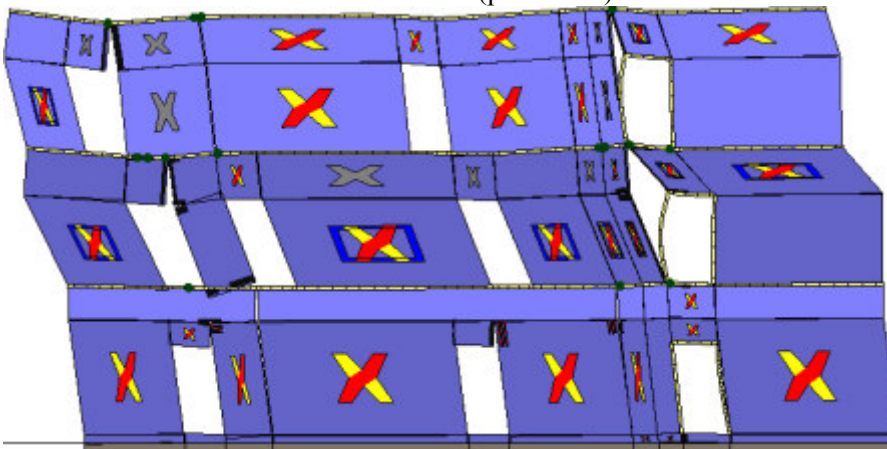
Analisi "Pushover -Y Acc". Configurazione della parete 21 in corrispondenza della capacità relativa allo stato limite SLV (passo 125).
