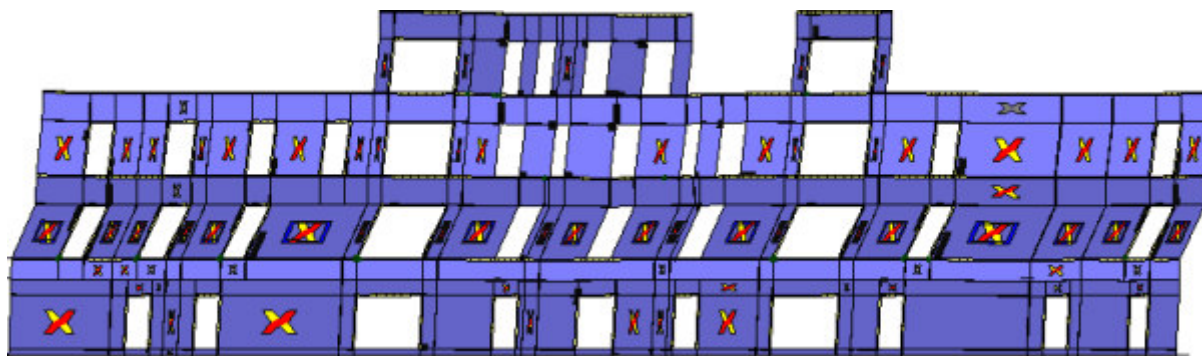
Analisi "Pushover +X Acc - e". Configurazione della parete 15 in corrispondenza della capacità relativa allo stato limite SLV (passo 86).
