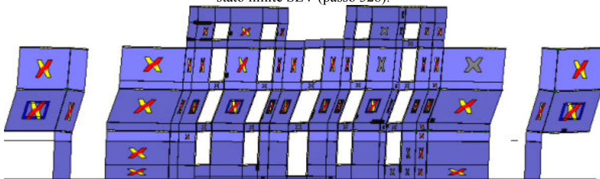
Analisi "Pushover +X Acc". Configurazione della parete 16 in corrispondenza della capacità relativa allo stato limite SLV (passo 328).
