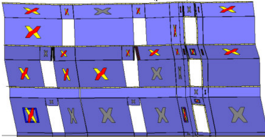
Analisi "Pushover -Y Massa + e". Configurazione della parete 32 in corrispondenza della capacità relativa allo stato limite SLV (passo 80).
