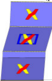
Analisi "Pushover +X Massa + e". Configurazione della parete 35 in corrispondenza della capacità relativa allo stato limite SLV (passo 83).
