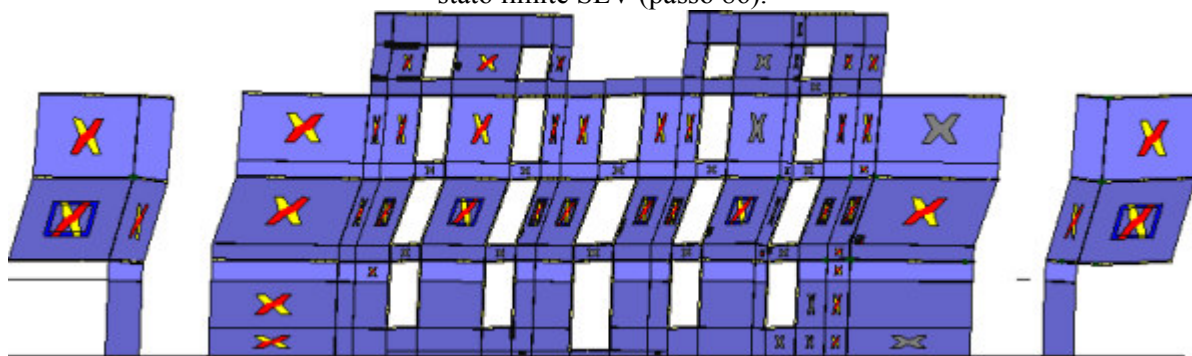
Analisi "Pushover +X Acc - e". Configurazione della parete 16 in corrispondenza della capacità relativa allo stato limite SLV (passo 86).
