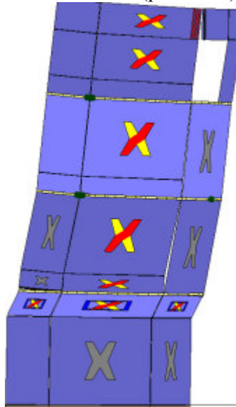
Analisi "Pushover +Y Acc - e". Configurazione della parete 4 in corrispondenza della capacità relativa allo stato limite SLV (passo 157).
