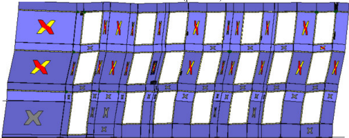
Analisi "Pushover +Y Acc - e". Configurazione della parete 34 in corrispondenza della capacità relativa allo stato limite SLV (passo 157).
