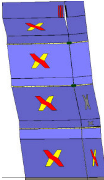
Analisi "Pushover +Y Acc - e". Configurazione della parete 2 in corrispondenza della capacità relativa allo stato limite SLV (passo 157).
