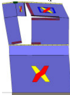
Analisi "Pushover -Y Acc + e". Configurazione della parete 14 in corrispondenza della capacità relativa allo stato limite SLV (passo 64).
