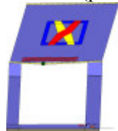
Analisi "Pushover +X Acc". Configurazione della parete 37 in corrispondenza della capacità relativa allo stato limite SLV (passo 328).
