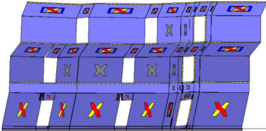
Analisi "Pushover +Y Acc + e". Configurazione della parete 32 in corrispondenza della capacità relativa allo stato limite SLV (passo 255).
