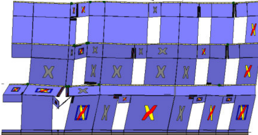
Analisi "Pushover +Y Massa + e". Configurazione della parete 18 in corrispondenza della capacità relativa allo stato limite SLV (passo 72).
