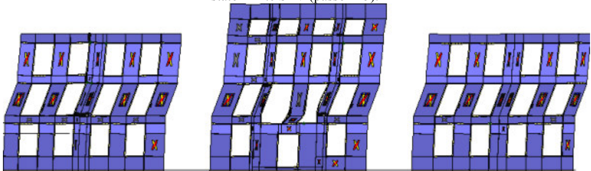
Analisi "Pushover +X Acc". Configurazione della parete 1 in corrispondenza della capacità relativa allo stato limite SLV (passo 328).
