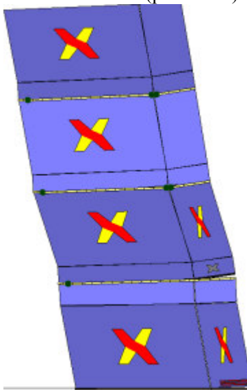
Analisi "Pushover +Y Acc + e". Configurazione della parete 5 in corrispondenza della capacità relativa allo stato limite SLV (passo 255).
