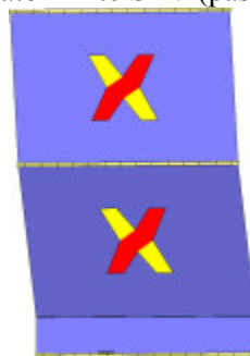
Analisi "Pushover -Y Massa + e". Configurazione della parete 23 in corrispondenza della capacità relativa allo stato limite SLV (passo 80).
