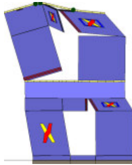
Analisi "Pushover -Y Acc". Configurazione della parete 13 in corrispondenza della capacità relativa allo stato limite SLV (passo 125).
