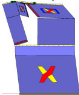
Analisi "Pushover -Y Acc". Configurazione della parete 14 in corrispondenza della capacità relativa allo stato limite SLV (passo 125).
