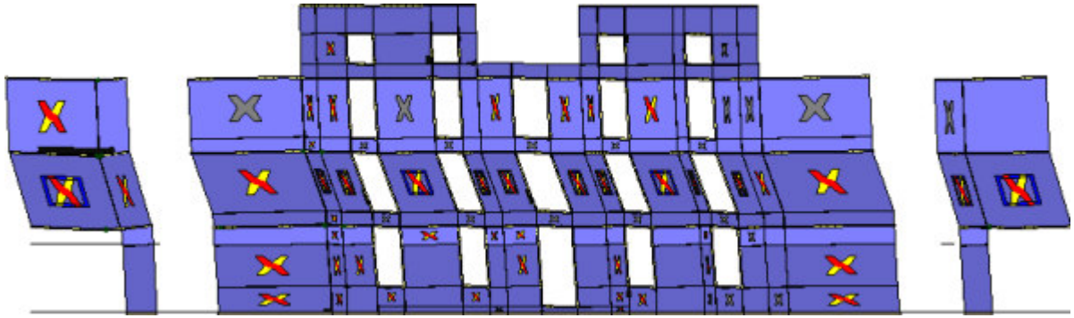
Analisi "Pushover -X Massa + e". Configurazione della parete 16 in corrispondenza della capacità relativa allo stato limite SLV (passo 79).
