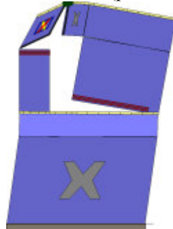
Analisi "Pushover +Y Acc - e". Configurazione della parete 14 in corrispondenza della capacità relativa allo stato limite SLV (passo 157).
