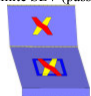
Analisi "Pushover -X Acc". Configurazione della parete 8 in corrispondenza della capacità relativa allo stato limite SLV (passo 299).
