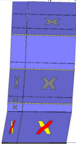
Analisi "Pushover +Y Massa - e". Configurazione della parete 6 in corrispondenza della capacità relativa allo stato limite SLV (passo 82).
