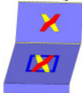
Analisi "Pushover +X Acc - e". Configurazione della parete 8 in corrispondenza della capacità relativa allo stato limite SLV (passo 86).
