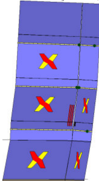
Analisi "Pushover -Y Massa". Configurazione della parete 5 in corrispondenza della capacità relativa allo stato limite SLV (passo 115).
