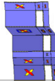
Analisi "Pushover -X Massa". Configurazione della parete 25 in corrispondenza della capacità relativa allo stato limite SLV (passo 79).
