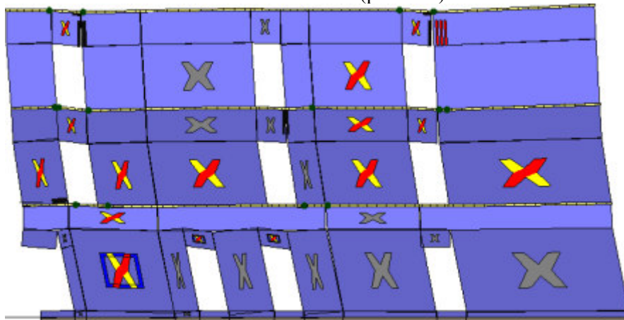
Analisi "Pushover -Y Massa + e". Configurazione della parete 33 in corrispondenza della capacità relativa allo stato limite SLV (passo 80).
