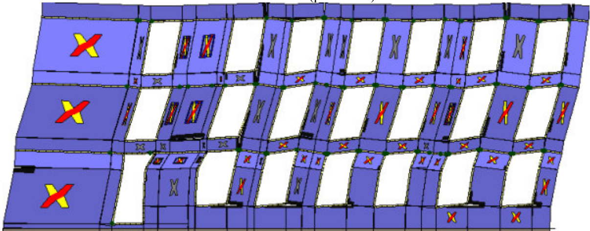
Analisi "Pushover +Y Acc + e". Configurazione della parete 7 in corrispondenza della capacità relativa allo stato limite SLV (passo 255).
