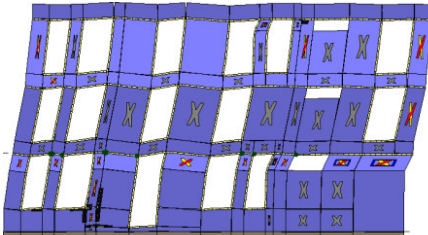
Analisi "Pushover +Y Acc - e". Configurazione della parete 22 in corrispondenza della capacità relativa allo stato limite SLV (passo 157).
