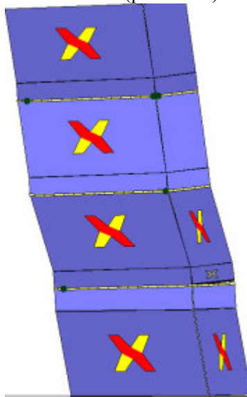
Analisi "Pushover +Y Acc". Configurazione della parete 5 in corrispondenza della capacità relativa allo stato
