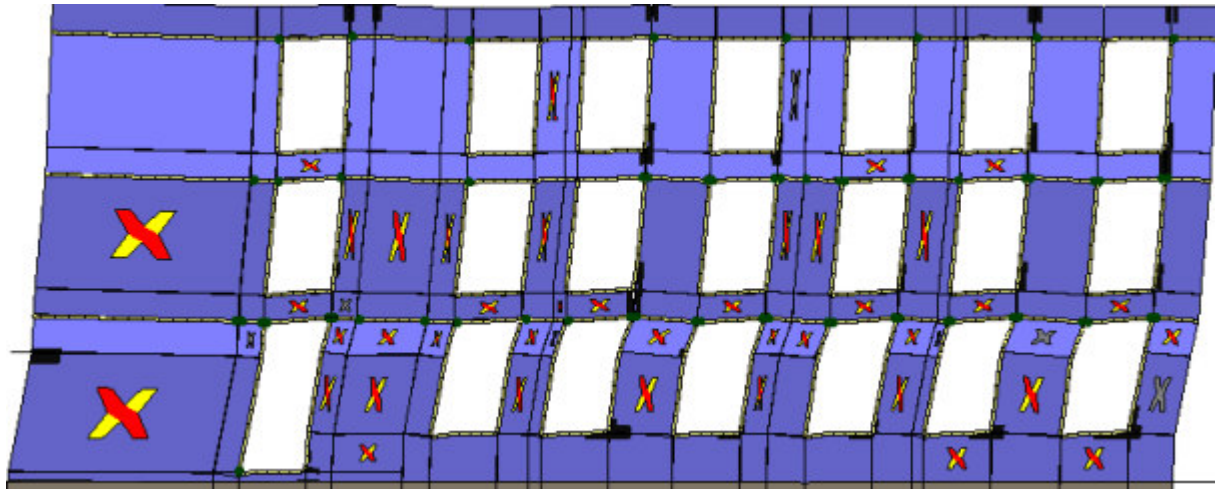
Analisi "Pushover +Y Massa". Configurazione della parete 34 in corrispondenza della capacità relativa allo stato limite SLV (passo 203).
