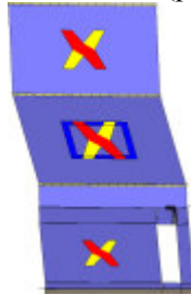
Analisi "Pushover -X Massa + e". Configurazione della parete 20 in corrispondenza della capacità relativa allo stato limite SLV (passo 79).
