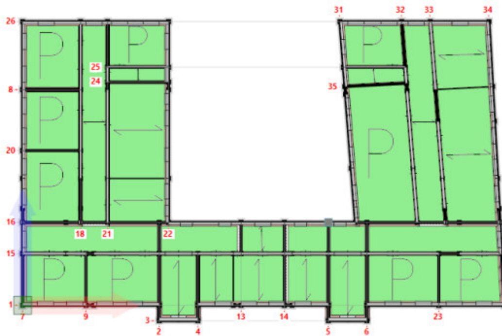
Pianta a quota 1480 cm con l'indicazione dei numeri attribuiti alle pareti.
