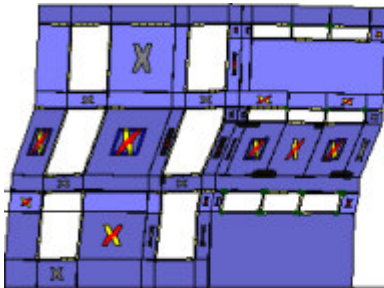
Analisi "Pushover +X Massa + e". Configurazione della parete 26 in corrispondenza della capacità relativa allo stato limite SLV (passo 83).
