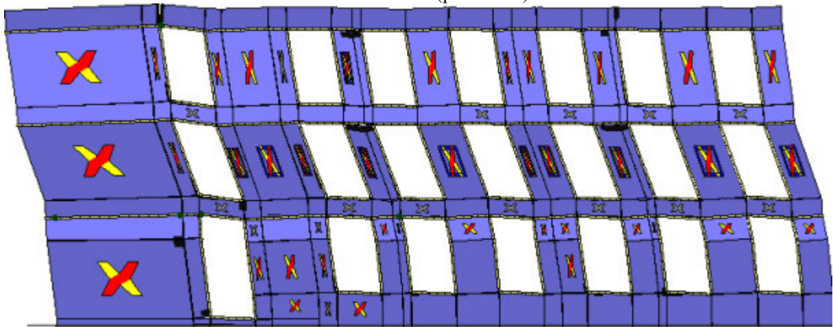
Analisi "Pushover -Y Acc". Configurazione della parete 34 in corrispondenza della capacità relativa allo stato limite SLV (passo 125).
