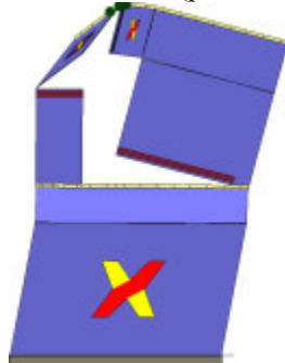
Analisi "Pushover +Y Acc + e". Configurazione della parete 14 in corrispondenza della capacità relativa allo stato limite SLV (passo 255).
