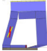
Analisi "Pushover -Y Massa + e". Configurazione della parete 30 in corrispondenza della capacità relativa allo stato limite SLV (passo 80).
