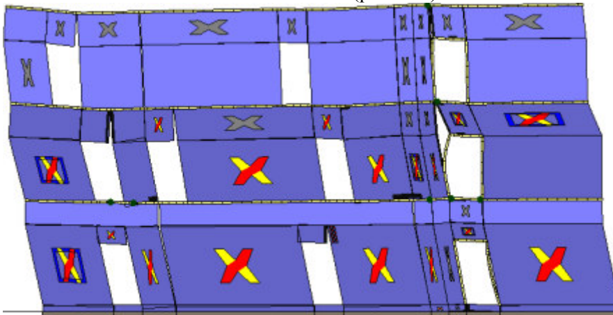
Analisi "Pushover -Y Massa - e". Configurazione della parete 21 in corrispondenza della capacità relativa allo stato limite SLV (passo 78).
