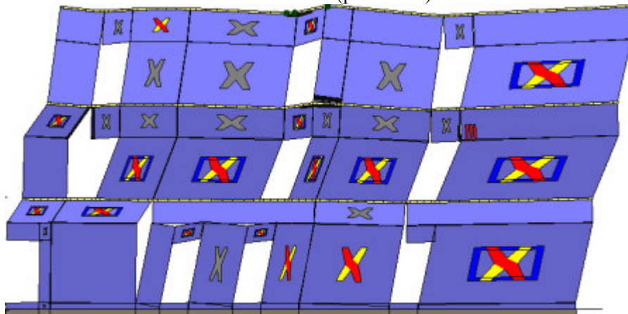
Analisi "Pushover +Y Acc". Configurazione della parete 33 in corrispondenza della capacità relativa allo stato limite SLV (passo 228).
