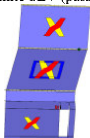
Analisi "Pushover +X Acc". Configurazione della parete 20 in corrispondenza della capacità relativa allo stato limite SLV (passo 328).
