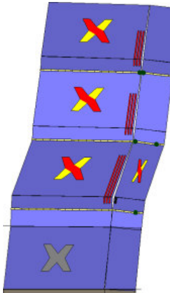
Analisi "Pushover -Y Acc - e". Configurazione della parete 5 in corrispondenza della capacità relativa allo stato limite SLV (passo 204).
