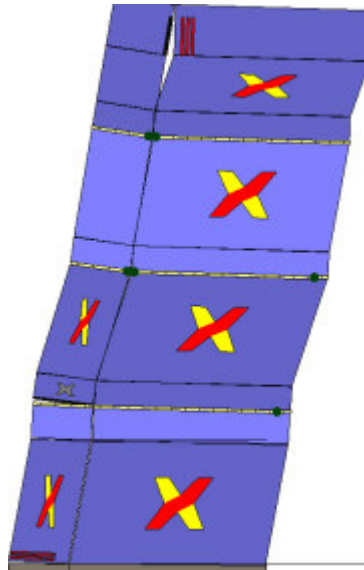
Analisi "Pushover +Y Acc + e". Configurazione della parete 6 in corrispondenza della capacità relativa allo stato limite SLV (passo 255).
