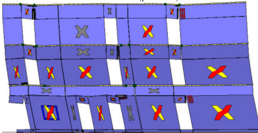
Analisi "Pushover -Y Massa". Configurazione della parete 33 in corrispondenza della capacità relativa allo stato limite SLV (passo 115).
