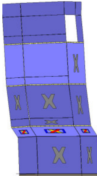
Analisi "Pushover -Y Massa + e". Configurazione della parete 4 in corrispondenza della capacità relativa allo stato limite SLV (passo 80).
