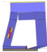
Analisi "Pushover -Y Massa - e". Configurazione della parete 30 in corrispondenza della capacità relativa allo stato limite SLV (passo 78).
