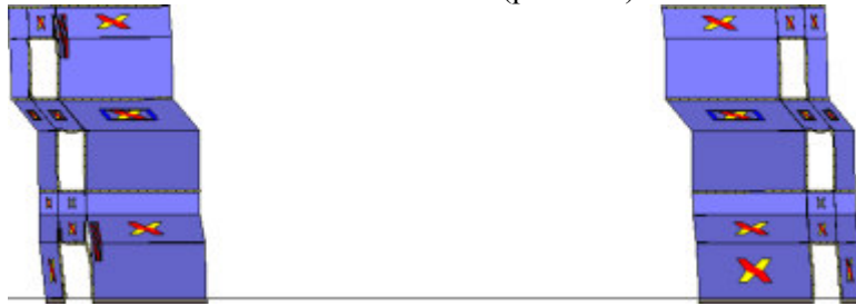
Analisi "Pushover -X Massa - e". Configurazione della parete 25 in corrispondenza della capacità relativa allo stato limite SLV (passo 79).
