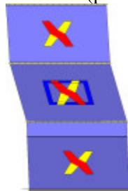
Analisi "Pushover -X Acc". Configurazione della parete 35 in corrispondenza della capacità relativa allo stato limite SLV (passo 299).
