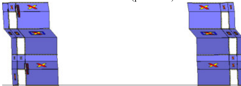
Analisi "Pushover -X Acc". Configurazione della parete 25 in corrispondenza della capacità relativa allo stato limite SLV (passo 299).
