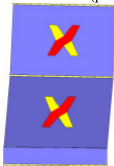
Analisi "Pushover +Y Massa + e". Configurazione della parete 23 in corrispondenza della capacità relativa allo stato limite SLV (passo 72).
