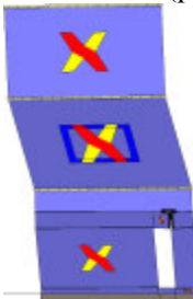
Analisi "Pushover -X Massa + e". Configurazione della parete 24 in corrispondenza della capacità relativa allo stato limite SLV (passo 79).
