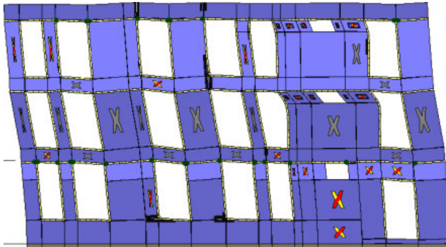
Analisi "Pushover -Y Acc + e". Configurazione della parete 31 in corrispondenza della capacità relativa allo stato limite SLV (passo 64).
