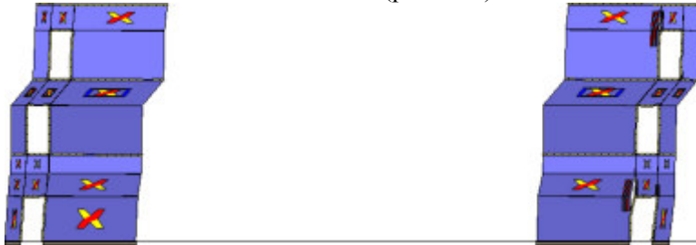
Analisi "Pushover +X Massa". Configurazione della parete 25 in corrispondenza della capacità relativa allo stato limite SLV (passo 84).
