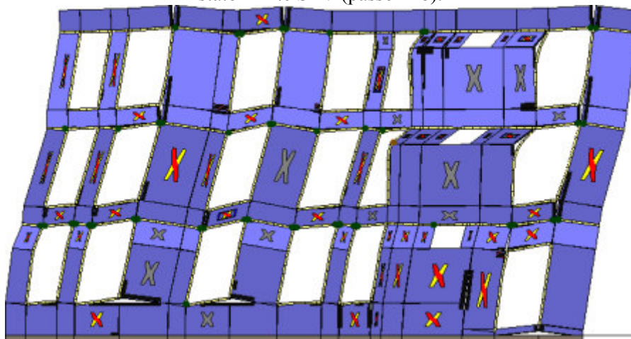
Analisi "Pushover +Y Acc". Configurazione della parete 31 in corrispondenza della capacità relativa allo stato limite SLV (passo 228).
