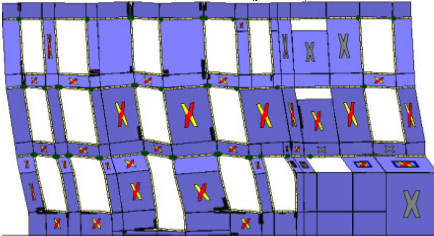
Analisi "Pushover -Y Massa - e". Configurazione della parete 22 in corrispondenza della capacità relativa allo stato limite SLV (passo 78).
