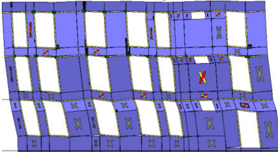
Analisi "Pushover -Y Massa + e". Configurazione della parete 31 in corrispondenza della capacità relativa allo stato limite SLV (passo 80).
