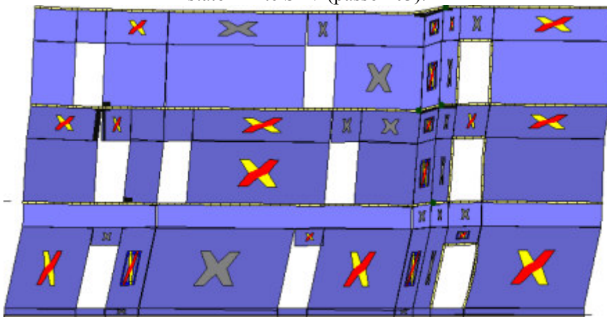
Analisi "Pushover +Y Massa". Configurazione della parete 21 in corrispondenza della capacità relativa allo stato limite SLV (passo 203).
