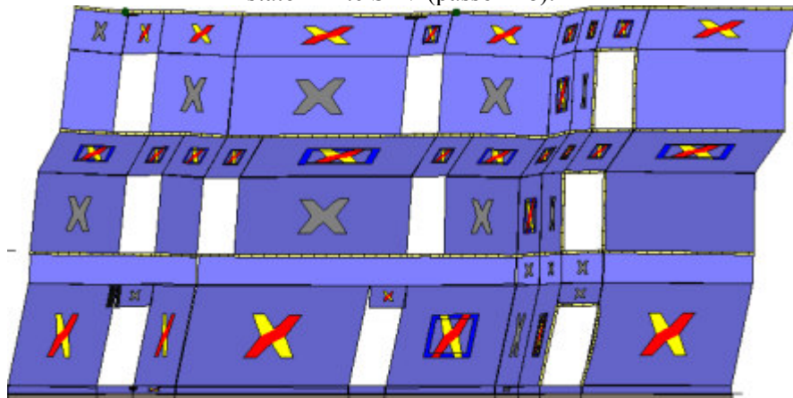
Analisi "Pushover +Y Acc". Configurazione della parete 21 in corrispondenza della capacità relativa allo stato limite SLV (passo 228).
