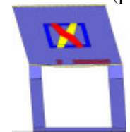
Analisi "Pushover -X Massa - e". Configurazione della parete 37 in corrispondenza della capacità relativa allo stato limite SLV (passo 79).
