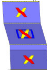
Analisi "Pushover -X Acc - e". Configurazione della parete 35 in corrispondenza della capacità relativa allo stato limite SLV (passo 134).
