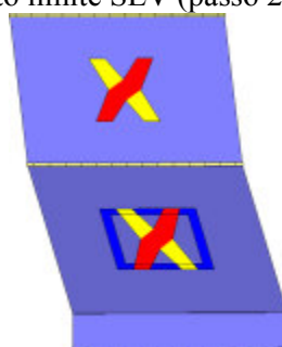
Analisi "Pushover -Y Acc - e". Configurazione della parete 23 in corrispondenza della capacità relativa allo stato limite SLV (passo 204).
