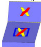
Analisi "Pushover +X Acc + e". Configurazione della parete 8 in corrispondenza della capacità relativa allo stato limite SLV (passo 86).
