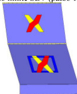
Analisi "Pushover -Y Acc". Configurazione della parete 34 in corrispondenza della capacità relativa allo stato limite SLV (passo 125).
