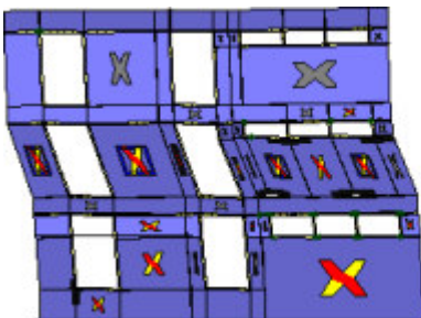
Analisi "Pushover -X Massa". Configurazione della parete 25 in corrispondenza della capacità relativa allo stato limite SLV (passo 79).
