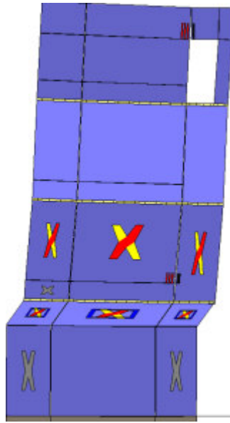
Analisi "Pushover +Y Massa + e". Configurazione della parete 4 in corrispondenza della capacità relativa allo stato limite SLV (passo 72).
