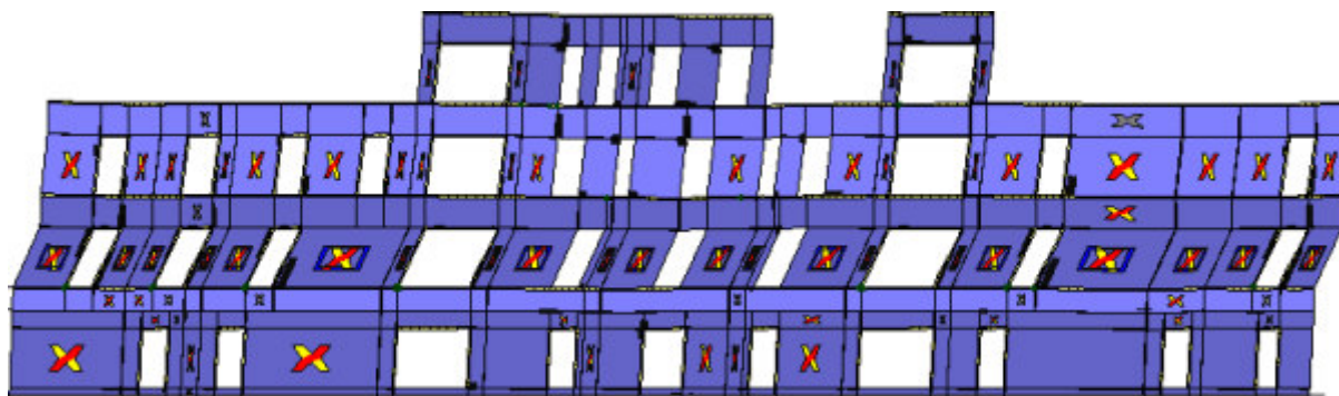
Analisi "Pushover +X Acc". Configurazione della parete 15 in corrispondenza della capacità relativa allo stato limite SLV (passo 328).
