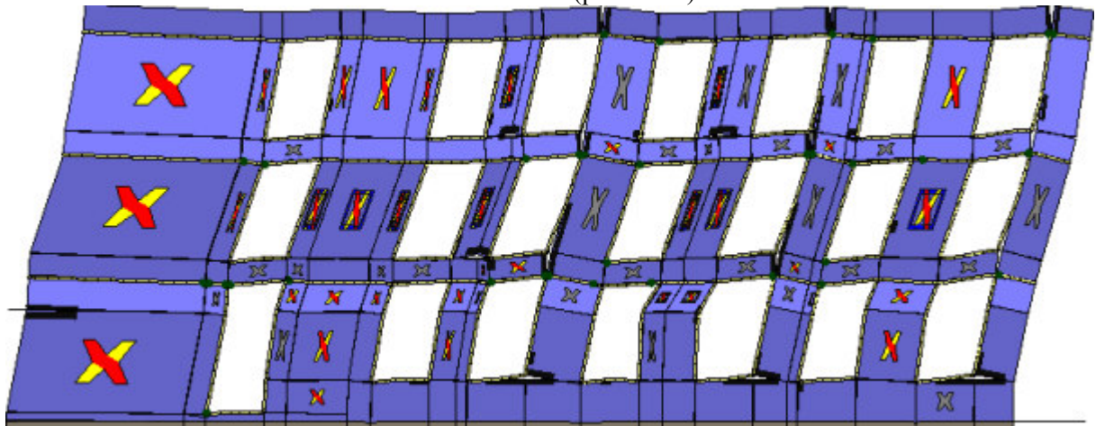
Analisi "Pushover +Y Acc + e". Configurazione della parete 34 in corrispondenza della capacità relativa allo stato limite SLV (passo 255).
