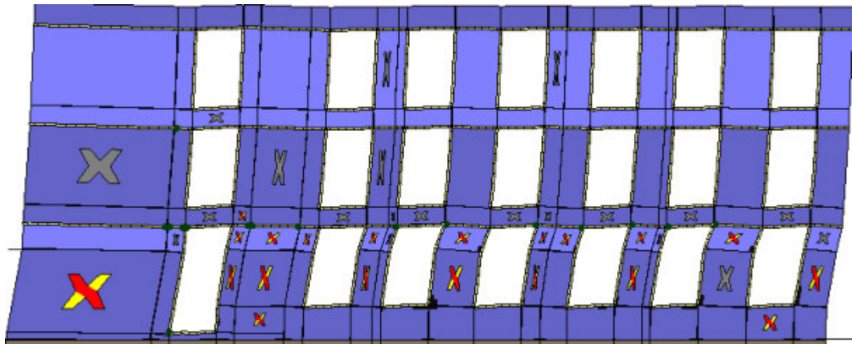
Analisi "Pushover +Y Massa - e". Configurazione della parete 34 in corrispondenza della capacità relativa allo stato limite SLV (passo 82).
