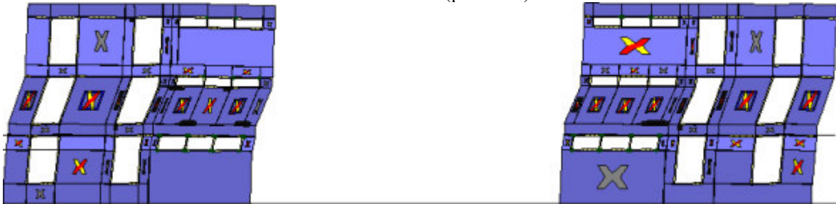
Analisi "Pushover +X Massa". Configurazione della parete 26 in corrispondenza della capacità relativa allo stato limite SLV (passo 84).
