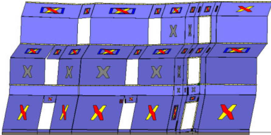
Analisi "Pushover +Y Acc". Configurazione della parete 32 in corrispondenza della capacità relativa allo stato limite SLV (passo 228).
