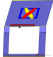
Analisi "Pushover +X Acc - e". Configurazione della parete 37 in corrispondenza della capacità relativa allo stato limite SLV (passo 86).
