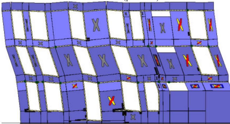
Analisi "Pushover -Y Acc - e". Configurazione della parete 22 in corrispondenza della capacità relativa allo stato limite SLV (passo 204).
