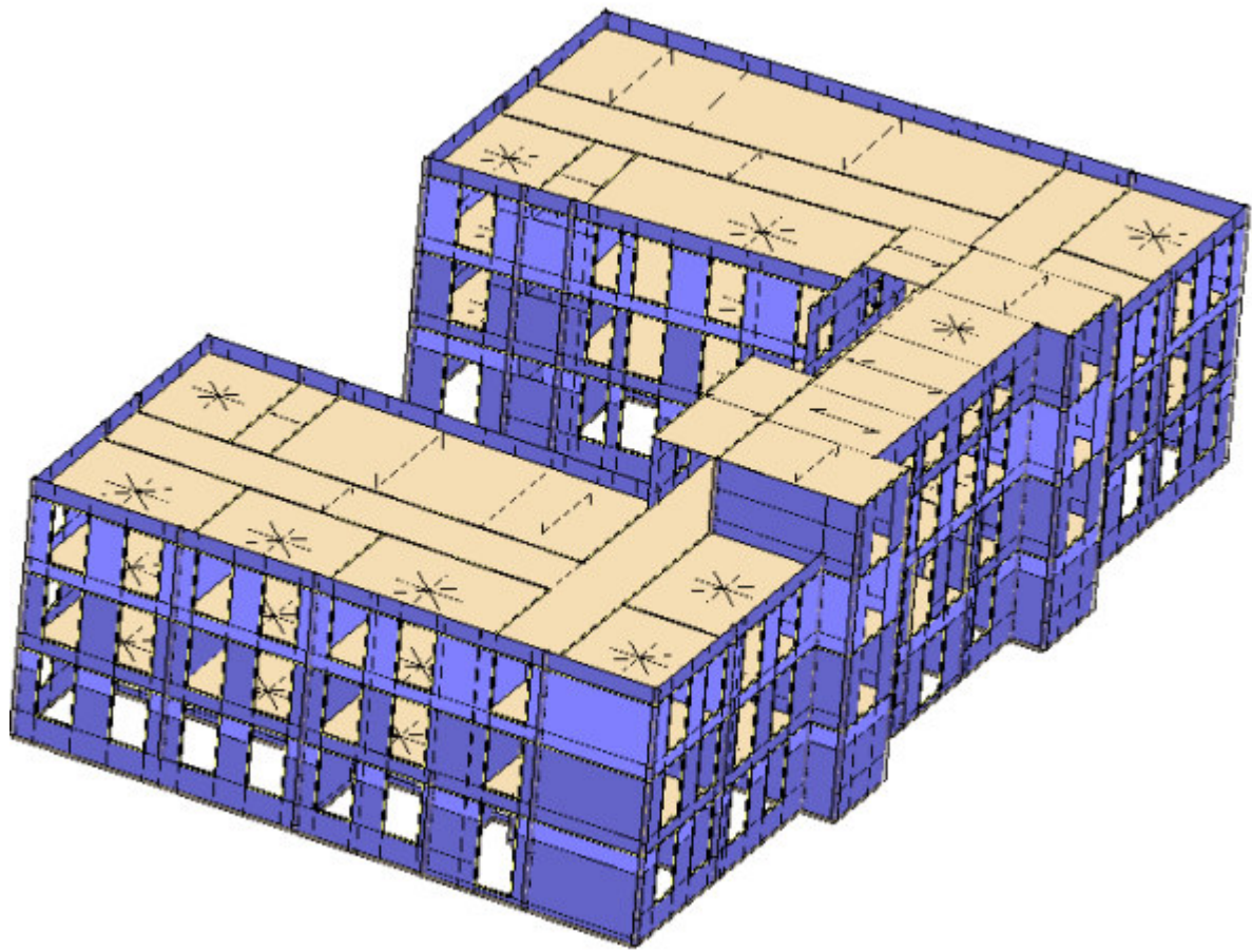
Modello 3DMacro - Vista assometrica 1.
