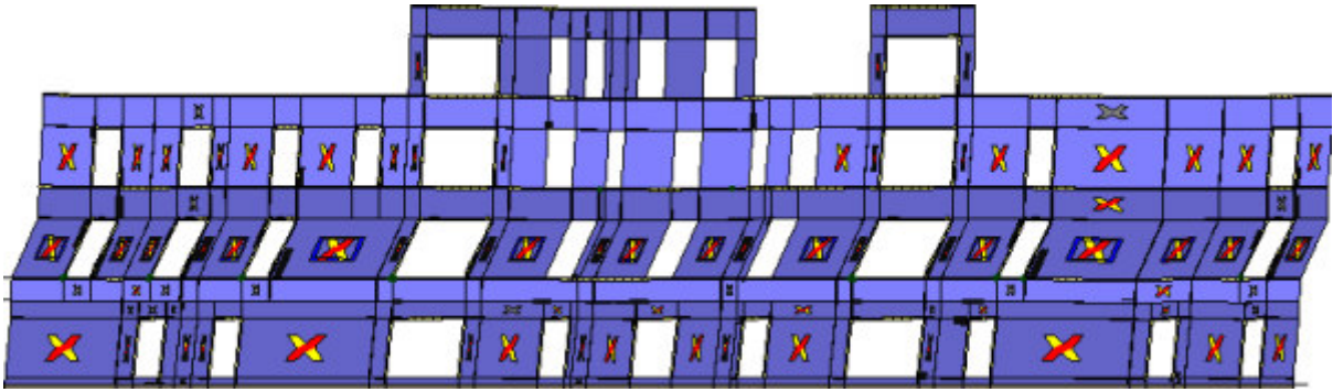
Analisi "Pushover +X Massa - e". Configurazione della parete 15 in corrispondenza della capacità relativa allo stato limite SLV (passo 84).
