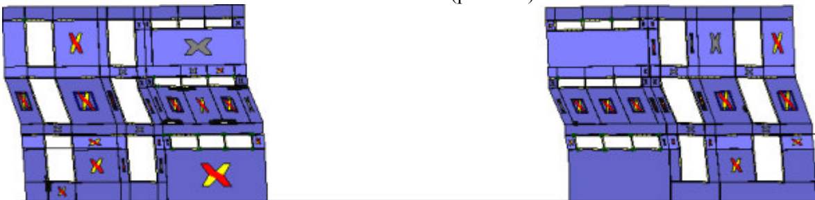
Analisi "Pushover -X Massa + e". Configurazione della parete 25 in corrispondenza della capacità relativa allo stato limite SLV (passo 79).
