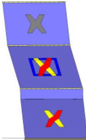
Analisi "Pushover -Y Acc - e". Configurazione della parete 9 in corrispondenza della capacità relativa allo stato limite SLV (passo 204).
