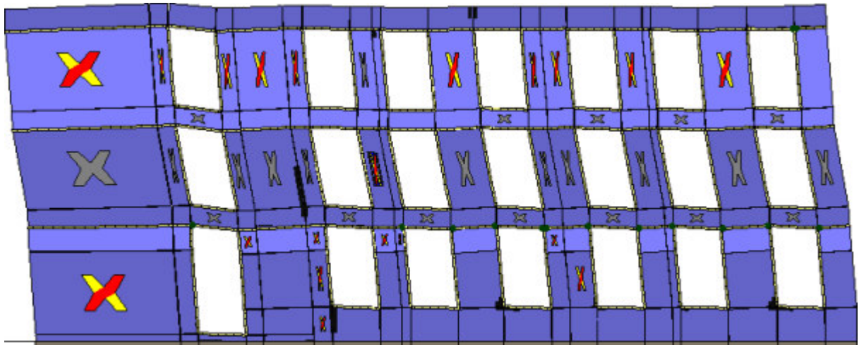
Analisi "Pushover -Y Acc + e". Configurazione della parete 34 in corrispondenza della capacità relativa allo stato limite SLV (passo 64).
