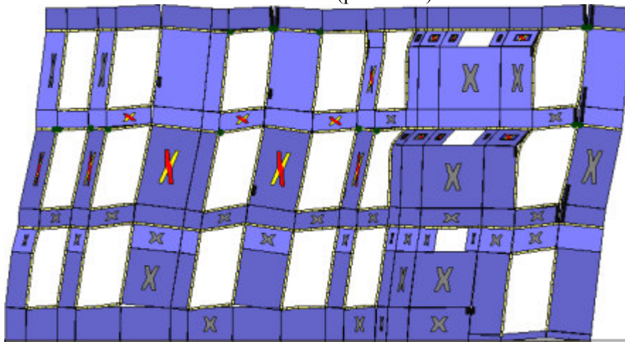
Analisi "Pushover +Y Acc - e". Configurazione della parete 31 in corrispondenza della capacità relativa allo stato limite SLV (passo 157).
