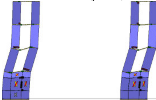
Analisi "Pushover +X Massa". Configurazione della parete 3 in corrispondenza della capacità relativa allo stato limite SLV (passo 84).
