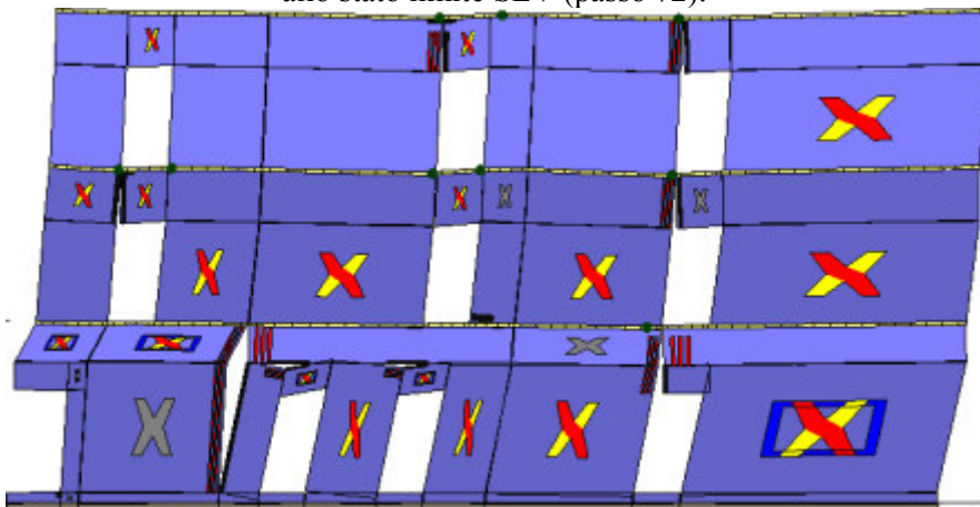
Analisi "Pushover +Y Massa + e". Configurazione della parete 33 in corrispondenza della capacità relativa allo stato limite SLV (passo 72).
