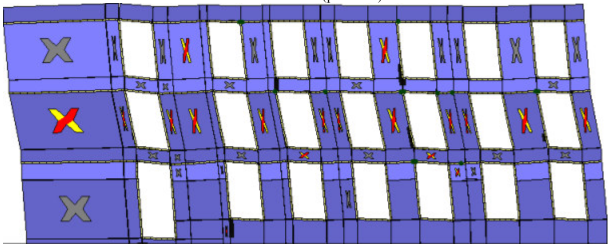
Analisi "Pushover -Y Acc + e". Configurazione della parete 7 in corrispondenza della capacità relativa allo stato limite SLV (passo 64).
