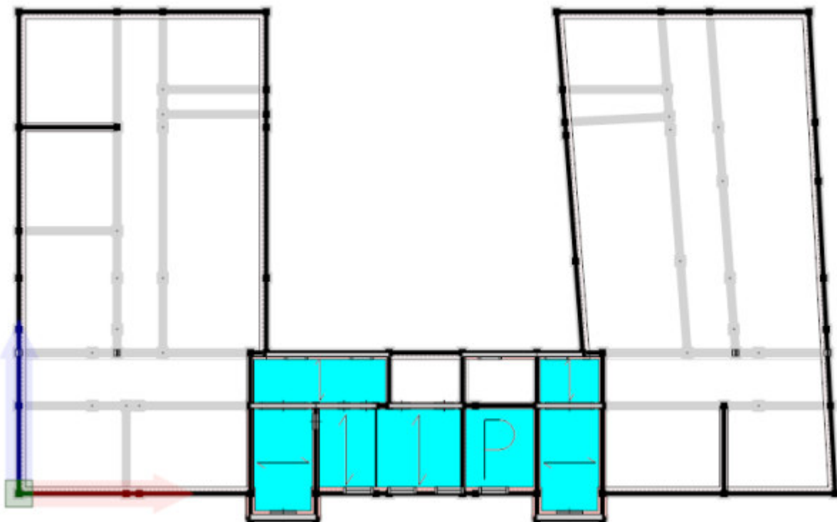
Pianta a quota 1480 cm: carichi di area applicati ai solai.
