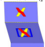
Analisi "Pushover -X Massa - e". Configurazione della parete 8 in corrispondenza della capacità relativa allo stato limite SLV (passo 79).
