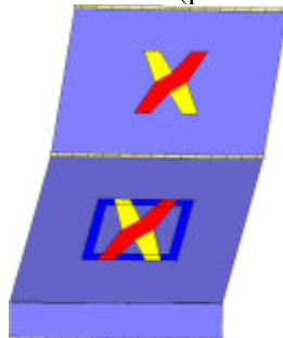
Analisi "Pushover +Y Acc + e". Configurazione della parete 23 in corrispondenza della capacità relativa allo stato limite SLV (passo 255).
