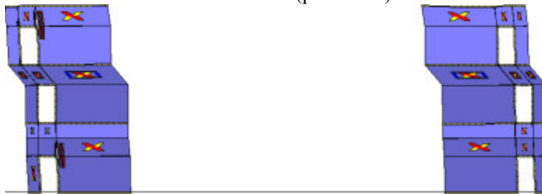
Analisi "Pushover -X Acc - e". Configurazione della parete 25 in corrispondenza della capacità relativa allo stato limite SLV (passo 134).
