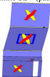
Analisi "Pushover +X Acc + e". Configurazione della parete 20 in corrispondenza della capacità relativa allo stato limite SLV (passo 86).
