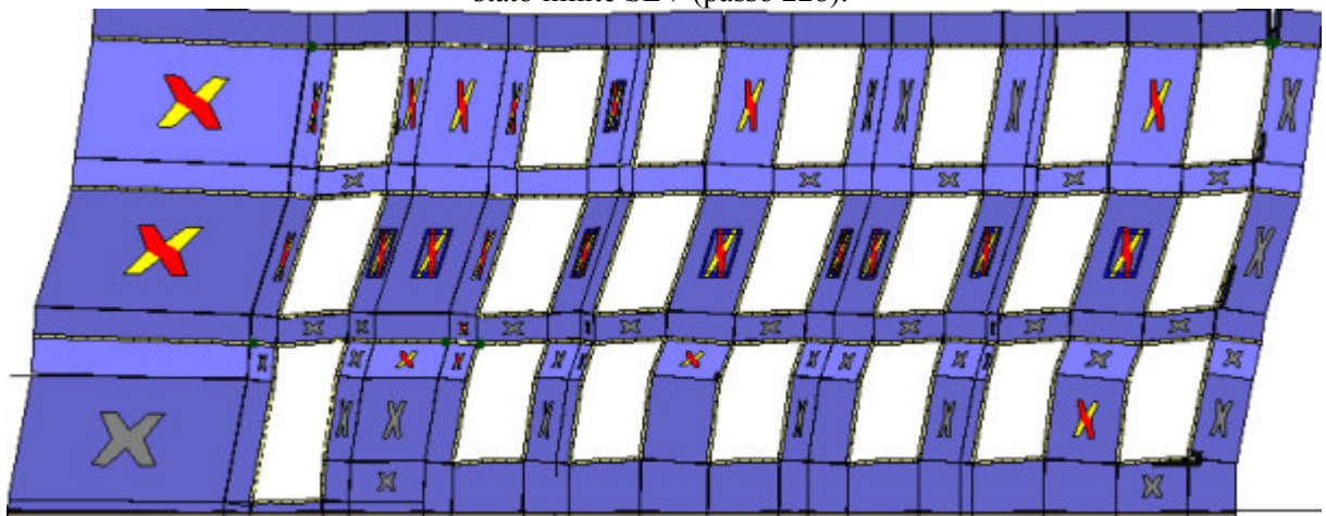
Analisi "Pushover +Y Acc". Configurazione della parete 34 in corrispondenza della capacità relativa allo stato limite SLV (passo 228).
