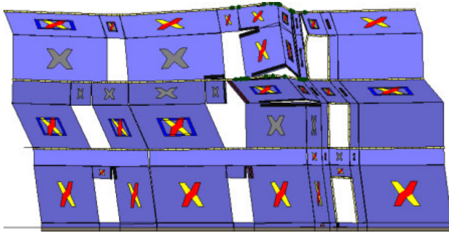
Analisi "Pushover -Y Acc". Configurazione della parete 32 in corrispondenza della capacità relativa allo stato limite SLV (passo 125).
