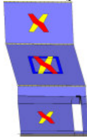
Analisi "Pushover -X Massa". Configurazione della parete 20 in corrispondenza della capacità relativa allo stato limite SLV (passo 79).
