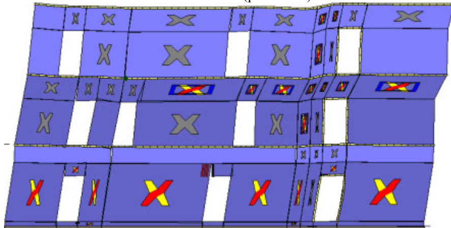
Analisi "Pushover +Y Acc - e". Configurazione della parete 21 in corrispondenza della capacità relativa allo stato limite SLV (passo 157).
