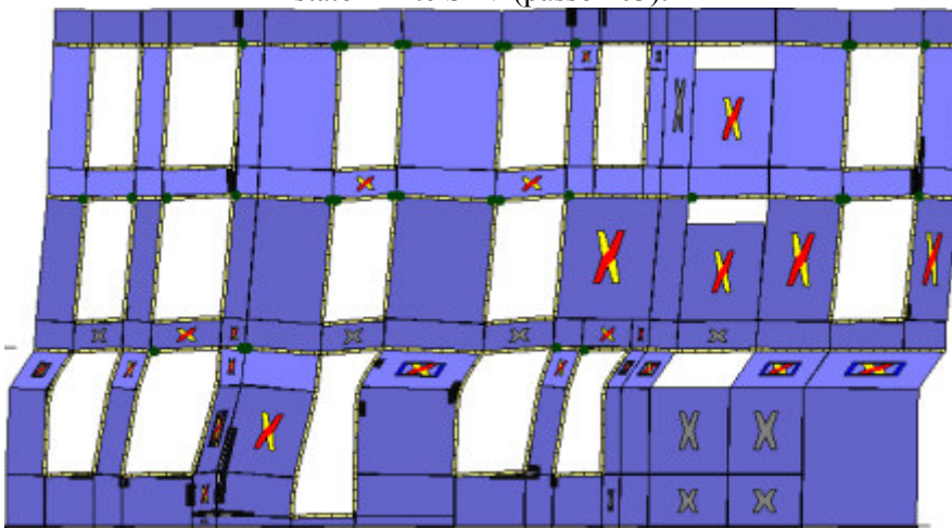
Analisi "Pushover +Y Massa". Configurazione della parete 22 in corrispondenza della capacità relativa allo stato limite SLV (passo 203).
