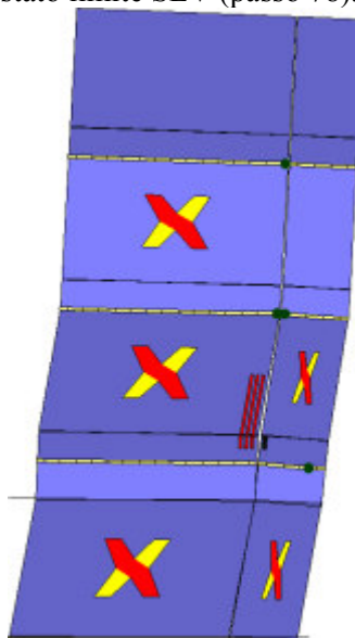
Analisi "Pushover -Y Massa - e". Configurazione della parete 5 in corrispondenza della capacità relativa allo stato limite SLV (passo 78).
