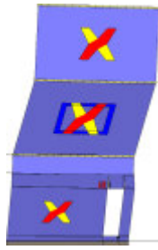
Analisi "Pushover +X Massa". Configurazione della parete 20 in corrispondenza della capacità relativa allo stato limite SLV (passo 84).
