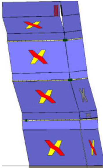
Analisi "Pushover +Y Acc". Configurazione della parete 2 in corrispondenza della capacità relativa allo stato limite SLV (passo 228).
