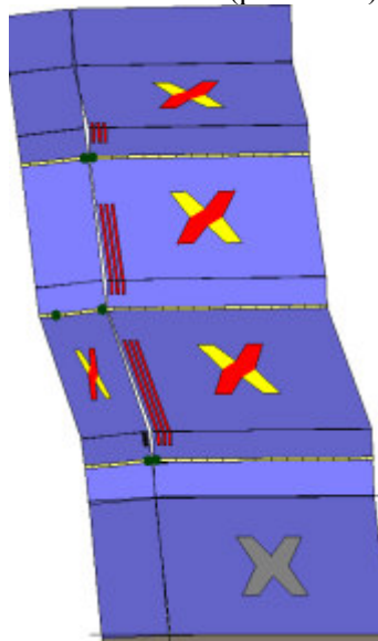
Analisi "Pushover -Y Acc - e". Configurazione della parete 6 in corrispondenza della capacità relativa allo stato limite SLV (passo 204).
