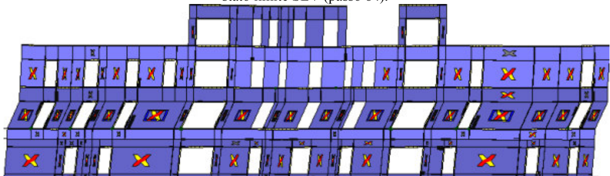
Analisi "Pushover +X Massa". Configurazione della parete 15 in corrispondenza della capacità relativa allo stato limite SLV (passo 84).
