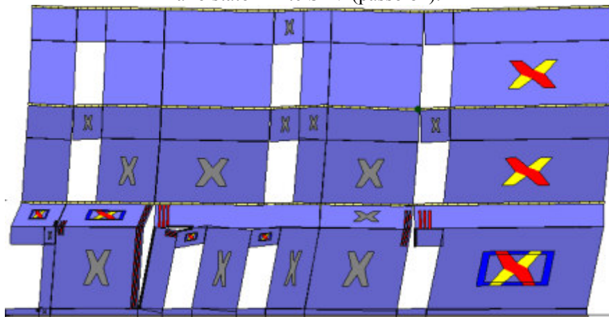
Analisi "Pushover +Y Massa - e". Configurazione della parete 33 in corrispondenza della capacità relativa allo stato limite SLV (passo 82).
