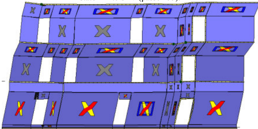
Analisi "Pushover +Y Acc + e". Configurazione della parete 21 in corrispondenza della capacità relativa allo stato limite SLV (passo 255).
