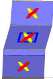
Analisi "Pushover +X Acc". Configurazione della parete 35 in corrispondenza della capacità relativa allo stato limite SLV (passo 328).
