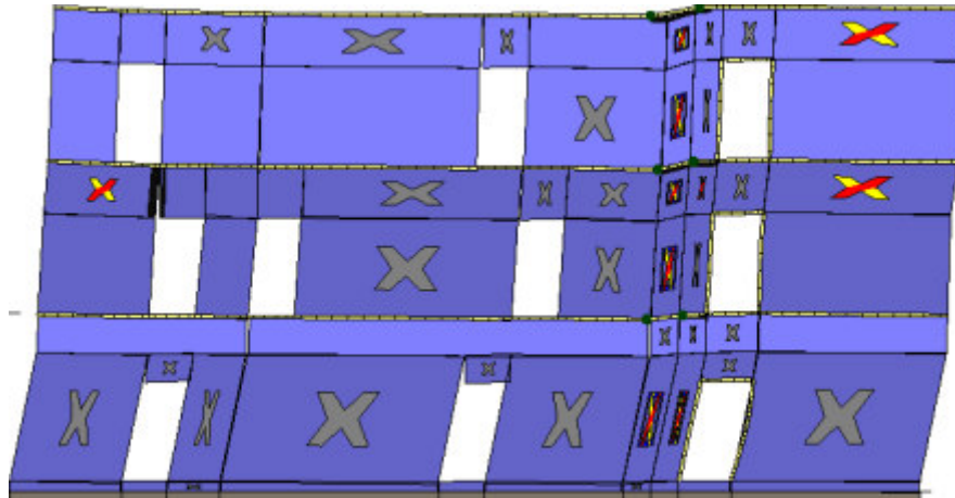
Analisi "Pushover +Y Massa - e". Configurazione della parete 21 in corrispondenza della capacità relativa allo stato limite SLV (passo 82).
