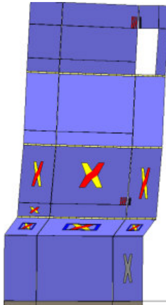
Analisi "Pushover +Y Massa". Configurazione della parete 4 in corrispondenza della capacità relativa allo stato limite SLV (passo 203).
