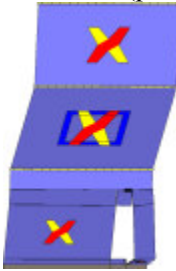
Analisi "Pushover +X Massa". Configurazione della parete 24 in corrispondenza della capacità relativa allo stato limite SLV (passo 84).
