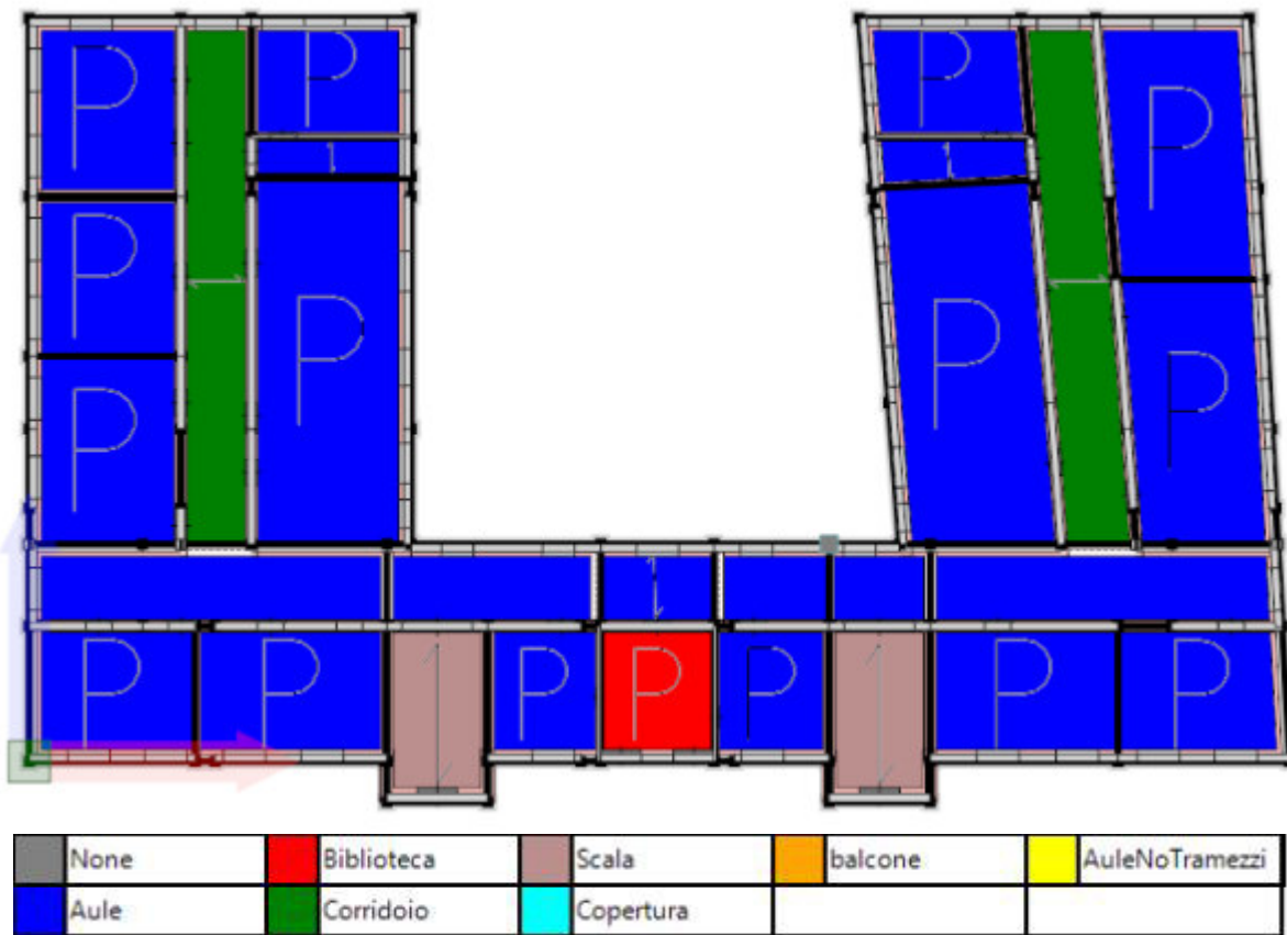
Pianta a quota 1040 cm: carichi di area applicati ai solai.
