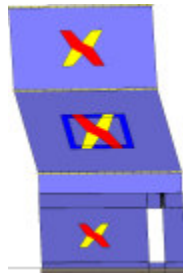
Analisi "Pushover -X Acc + e". Configurazione della parete 24 in corrispondenza della capacità relativa allo stato limite SLV (passo 135).
