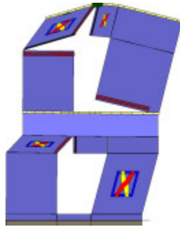
Analisi "Pushover +Y Acc". Configurazione della parete 13 in corrispondenza della capacità relativa allo stato limite SLV (passo 228).
