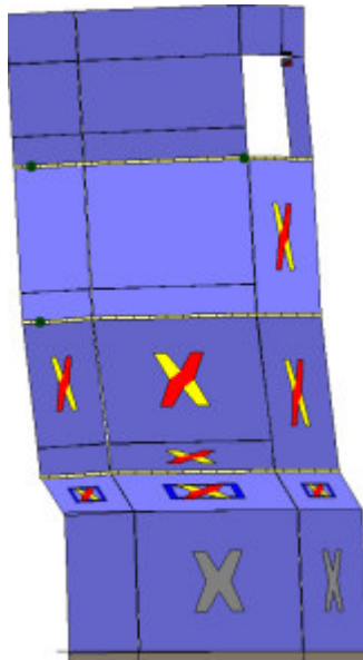
Analisi "Pushover -Y Massa". Configurazione della parete 4 in corrispondenza della capacità relativa allo stato limite SLV (passo 115).
