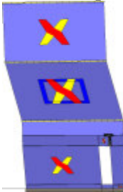
Analisi "Pushover -X Massa". Configurazione della parete 24 in corrispondenza della capacità relativa allo stato limite SLV (passo 79).
