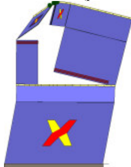
Analisi "Pushover +Y Acc". Configurazione della parete 14 in corrispondenza della capacità relativa allo stato limite SLV (passo 228).
