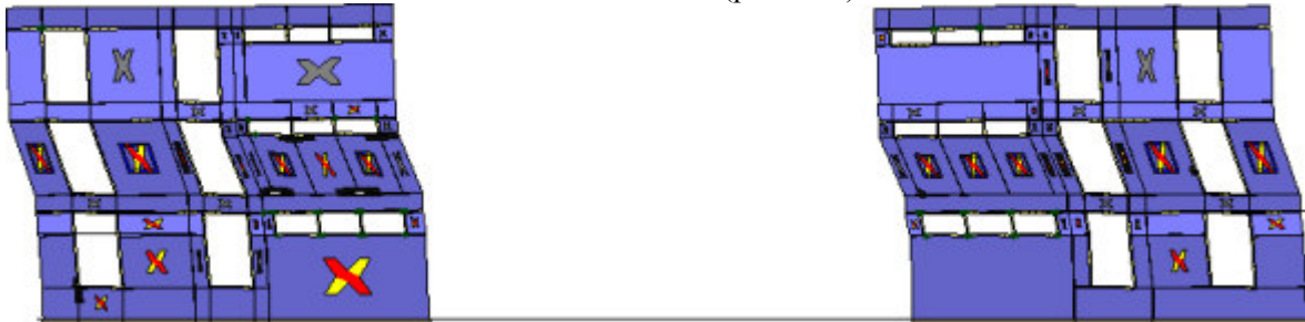
Analisi "Pushover -X Massa - e". Configurazione della parete 26 in corrispondenza della capacità relativa allo stato limite SLV (passo 79).
