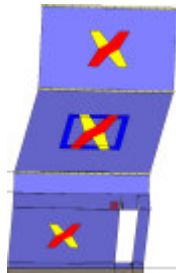
Analisi "Pushover +X Massa + e". Configurazione della parete 20 in corrispondenza della capacità relativa allo stato limite SLV (passo 83).
