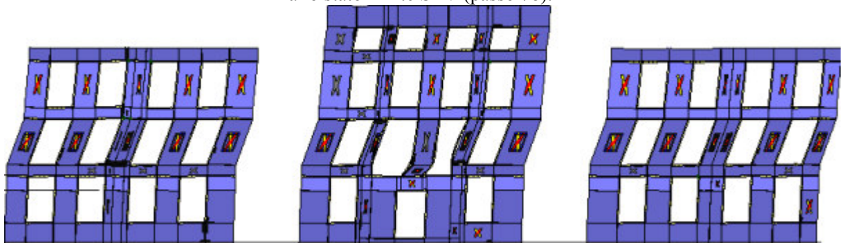
Analisi "Pushover +X Acc - e". Configurazione della parete 1 in corrispondenza della capacità relativa allo stato limite SLV (passo 86).
