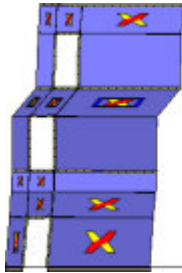
Analisi "Pushover +X Massa + e". Configurazione della parete 25 in corrispondenza della capacità relativa allo stato limite SLV (passo 83).
