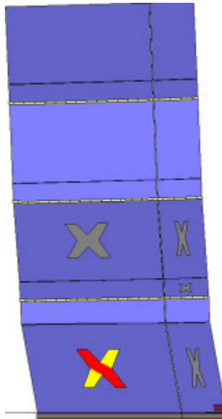
Analisi "Pushover +Y Massa - e". Configurazione della parete 5 in corrispondenza della capacità relativa allo stato limite SLV (passo 82).
