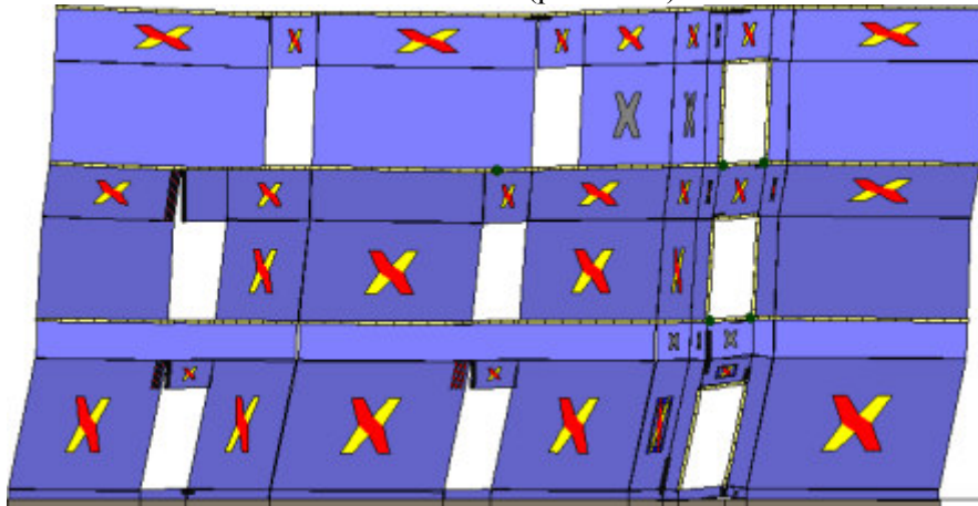
Analisi "Pushover +Y Massa". Configurazione della parete 32 in corrispondenza della capacità relativa allo stato limite SLV (passo 203).
