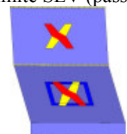
Analisi "Pushover -X Acc - e". Configurazione della parete 8 in corrispondenza della capacità relativa allo stato limite SLV (passo 134).
