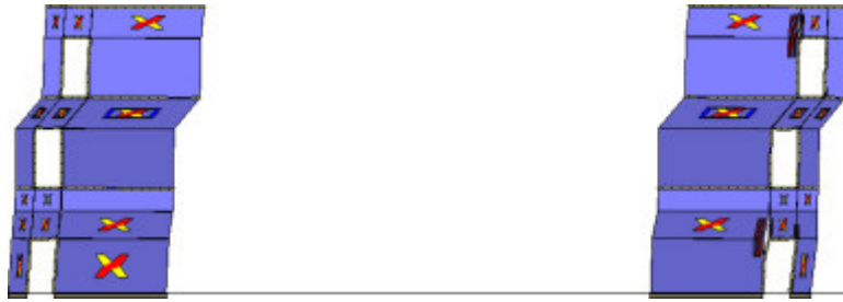
Analisi "Pushover +X Massa - e". Configurazione della parete 25 in corrispondenza della capacità relativa allo stato limite SLV (passo 84).
