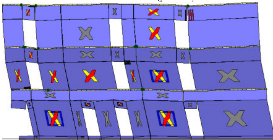
Analisi "Pushover -Y Massa - e". Configurazione della parete 33 in corrispondenza della capacità relativa allo stato limite SLV (passo 78).
