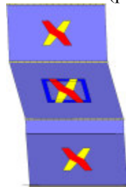
Analisi "Pushover -X Massa - e". Configurazione della parete 35 in corrispondenza della capacità relativa allo stato limite SLV (passo 79).
