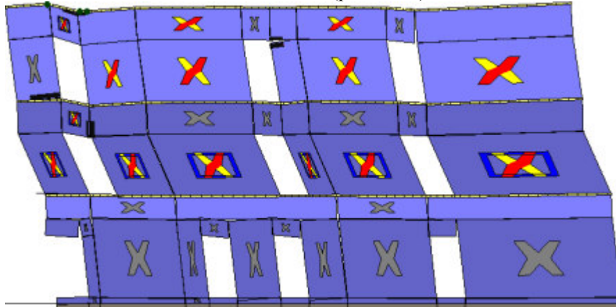
Analisi "Pushover -Y Acc - e". Configurazione della parete 33 in corrispondenza della capacità relativa allo stato limite SLV (passo 204).
