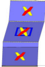
Analisi "Pushover +X Acc - e". Configurazione della parete 35 in corrispondenza della capacità relativa allo stato limite SLV (passo 86).
