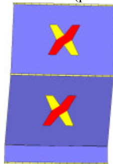
Analisi "Pushover +Y Massa". Configurazione della parete 23 in corrispondenza della capacità relativa allo stato limite SLV (passo 203).
