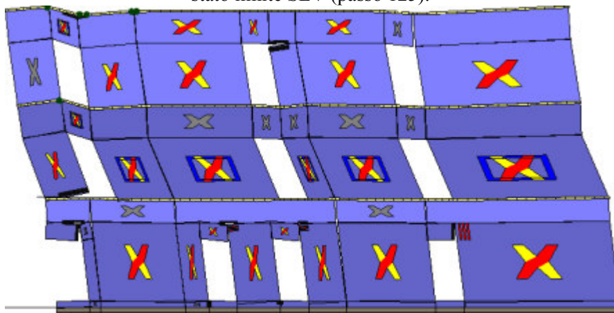
Analisi "Pushover -Y Acc". Configurazione della parete 33 in corrispondenza della capacità relativa allo stato limite SLV (passo 125).
