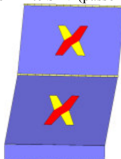
Analisi "Pushover +Y Acc - e". Configurazione della parete 34 in corrispondenza della capacità relativa allo stato limite SLV (passo 157).
