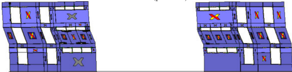
Analisi "Pushover -X Acc + e". Configurazione della parete 26 in corrispondenza della capacità relativa allo stato limite SLV (passo 135).
