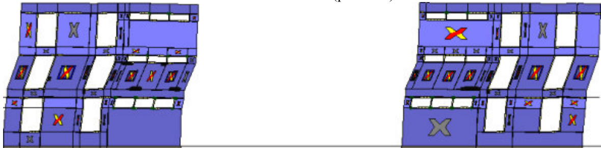
Analisi "Pushover +X Massa - e". Configurazione della parete 26 in corrispondenza della capacità relativa allo stato limite SLV (passo 84).
