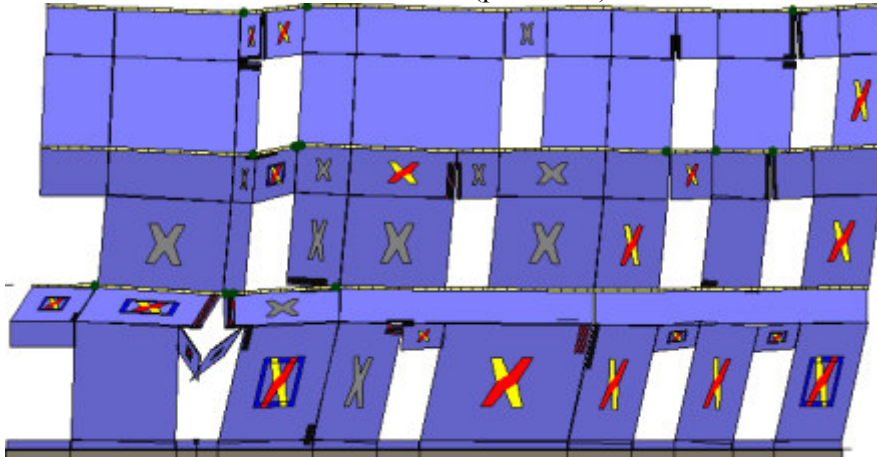
Analisi "Pushover +Y Massa". Configurazione della parete 18 in corrispondenza della capacità relativa allo stato limite SLV (passo 203).
