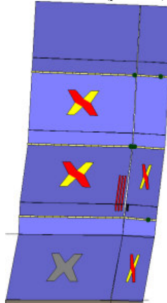
Analisi "Pushover -Y Massa + e". Configurazione della parete 5 in corrispondenza della capacità relativa allo stato limite SLV (passo 80).
