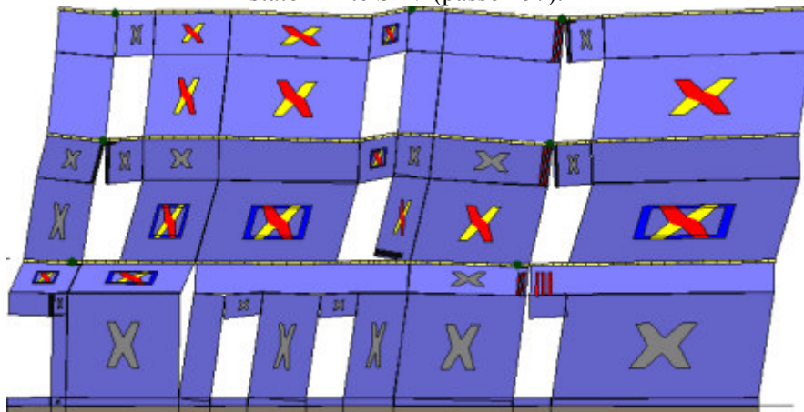
Analisi "Pushover +Y Acc - e". Configurazione della parete 33 in corrispondenza della capacità relativa allo stato limite SLV (passo 157).
