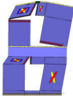
Analisi "Pushover +Y Acc - e". Configurazione della parete 13 in corrispondenza della capacità relativa allo stato limite SLV (passo 157).
