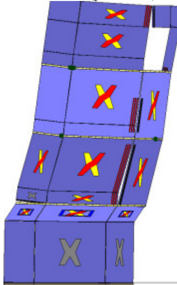
Analisi "Pushover +Y Acc". Configurazione della parete 4 in corrispondenza della capacità relativa allo stato limite SLV (passo 228).
