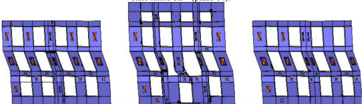
Analisi "Pushover +X Massa - e". Configurazione della parete 8 in corrispondenza della capacità relativa allo stato limite SLV (passo 84).
