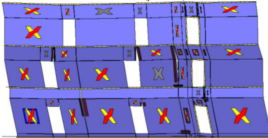
Analisi "Pushover -Y Massa". Configurazione della parete 32 in corrispondenza della capacità relativa allo stato limite SLV (passo 115).
