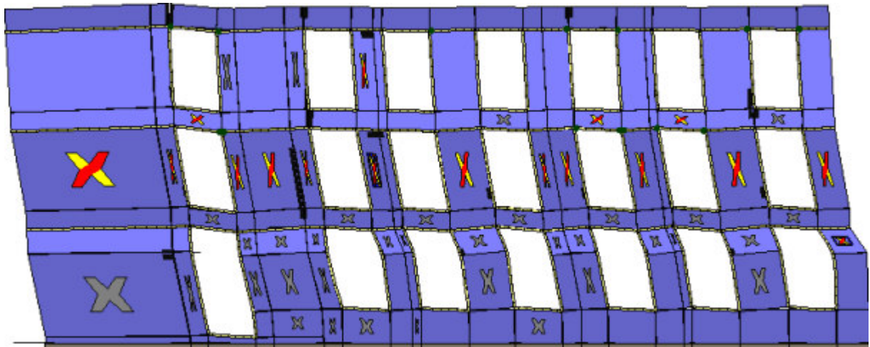
Analisi "Pushover -Y Massa - e". Configurazione della parete 34 in corrispondenza della capacità relativa allo stato limite SLV (passo 78).
