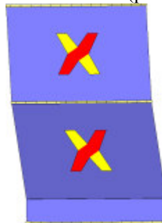
Analisi "Pushover -Y Massa - e". Configurazione della parete 23 in corrispondenza della capacità relativa allo stato limite SLV (passo 78).
