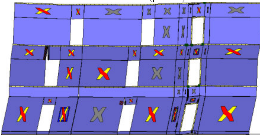
Analisi "Pushover +Y Massa + e". Configurazione della parete 32 in corrispondenza della capacità relativa allo stato limite SLV (passo 72).
