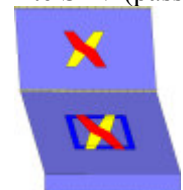
Analisi "Pushover -X Acc + e". Configurazione della parete 8 in corrispondenza della capacità relativa allo stato limite SLV (passo 135).
