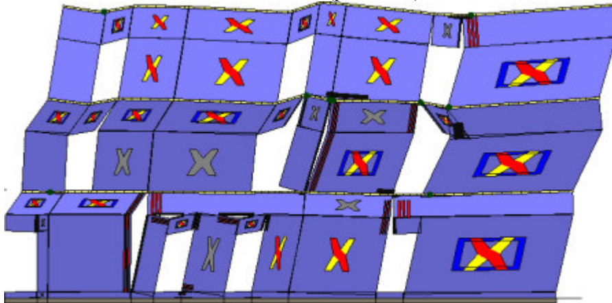
Analisi "Pushover +Y Acc + e". Configurazione della parete 33 in corrispondenza della capacità relativa allo stato limite SLV (passo 255).
