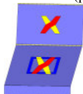
Analisi "Pushover +X Massa - e". Configurazione della parete 8 in corrispondenza della capacità relativa allo stato limite SLV (passo 84).
