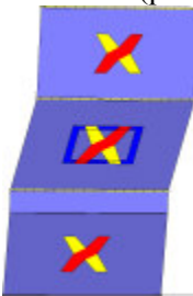
Analisi "Pushover +X Massa". Configurazione della parete 35 in corrispondenza della capacità relativa allo stato limite SLV (passo 84).
