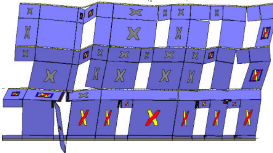
Analisi "Pushover +Y Acc - e". Configurazione della parete 18 in corrispondenza della capacità relativa allo stato limite SLV (passo 157).
