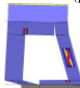
Analisi "Pushover -Y Massa - e". Configurazione della parete 29 in corrispondenza della capacità relativa allo stato limite SLV (passo 78).
