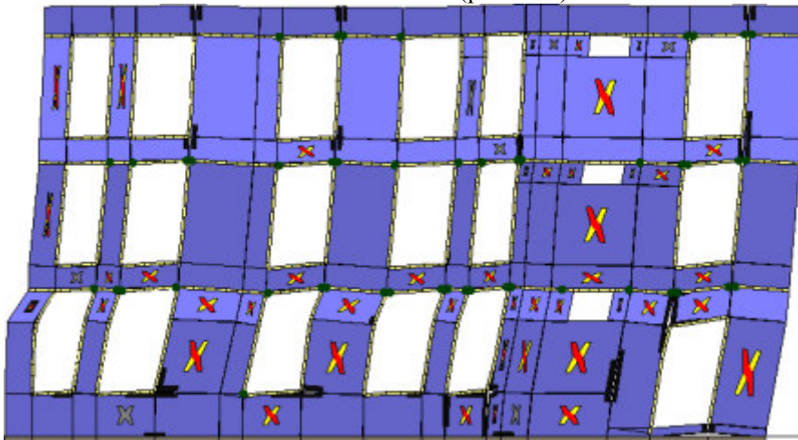
Analisi "Pushover +Y Massa + e". Configurazione della parete 31 in corrispondenza della capacità relativa allo stato limite SLV (passo 72).
