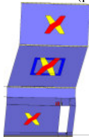
Analisi "Pushover +X Massa - e". Configurazione della parete 20 in corrispondenza della capacità relativa allo stato limite SLV (passo 84).
