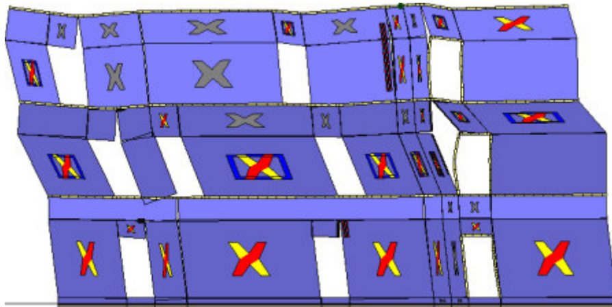
Analisi "Pushover -Y Acc - e". Configurazione della parete 21 in corrispondenza della capacità relativa allo stato limite SLV (passo 204).
