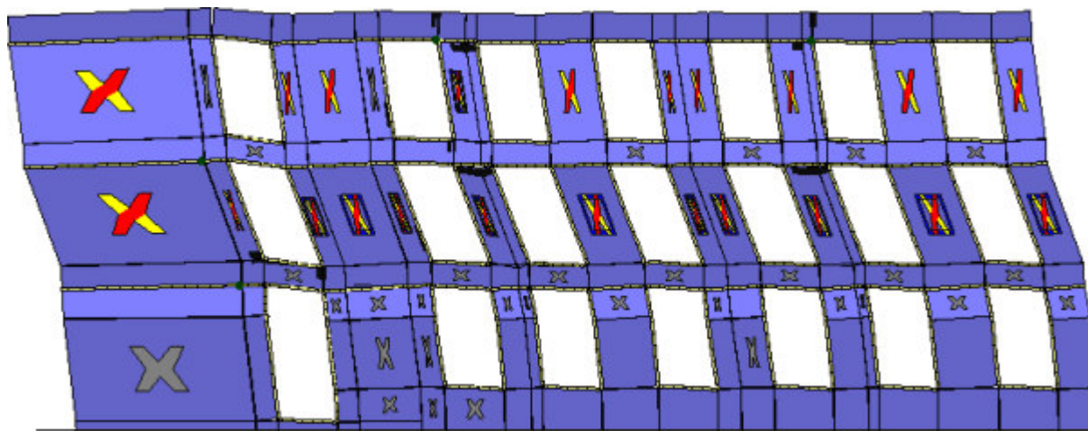
Analisi "Pushover -Y Acc - e". Configurazione della parete 34 in corrispondenza della capacità relativa allo stato limite SLV (passo 204).
