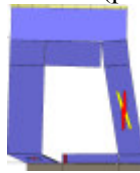
Analisi "Pushover -Y Acc". Configurazione della parete 29 in corrispondenza della capacità relativa allo stato limite SLV (passo 125).
