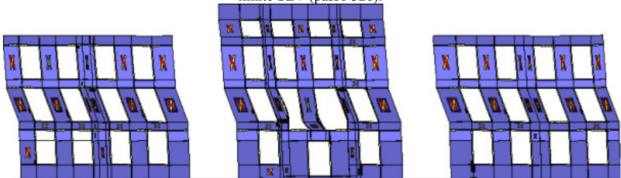
Analisi "Pushover +X Acc". Configurazione della parete 8 in corrispondenza della capacità relativa allo stato limite SLV (passo 328).
