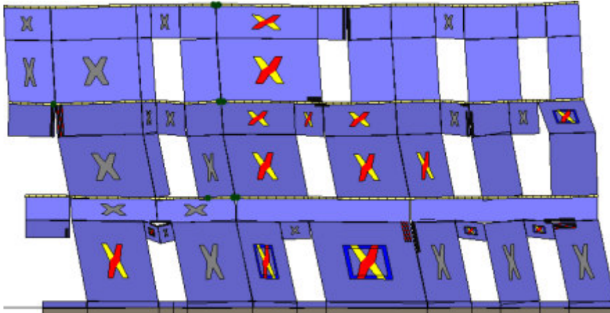
Analisi "Pushover -Y Massa - e". Configurazione della parete 18 in corrispondenza della capacità relativa allo stato limite SLV (passo 78).
