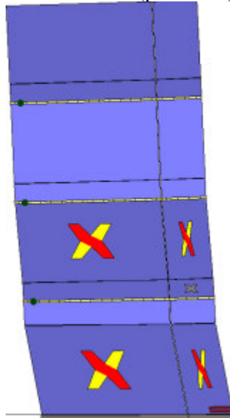
Analisi "Pushover +Y Massa". Configurazione della parete 5 in corrispondenza della capacità relativa allo stato limite SLV (passo 203).
