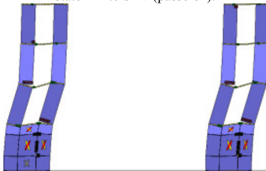
Analisi "Pushover +X Massa - e". Configurazione della parete 3 in corrispondenza della capacità relativa allo stato limite SLV (passo 84).
