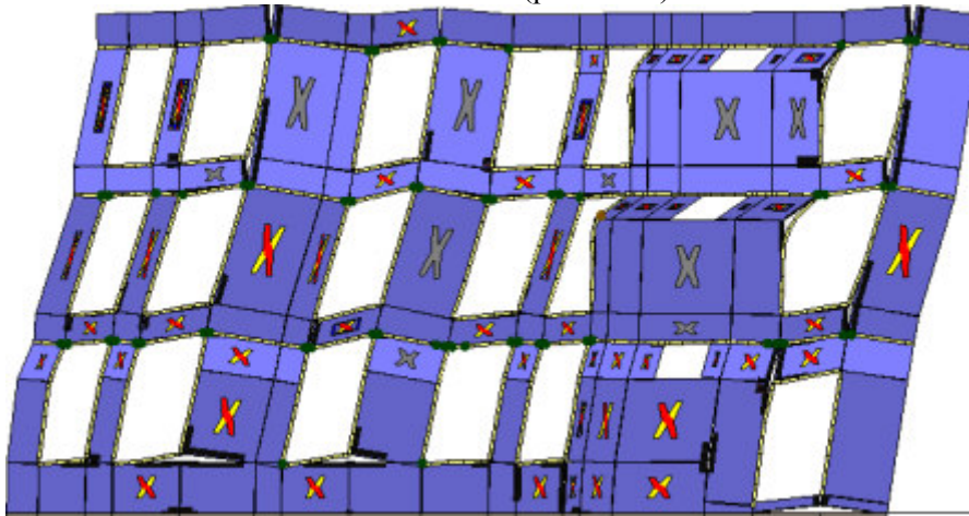
Analisi "Pushover +Y Acc + e". Configurazione della parete 31 in corrispondenza della capacità relativa allo stato limite SLV (passo 255).
