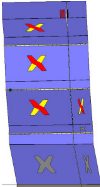
Analisi "Pushover +Y Massa - e". Configurazione della parete 2 in corrispondenza della capacità relativa allo stato limite SLV (passo 82).
