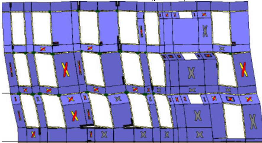
Analisi "Pushover -Y Massa - e". Configurazione della parete 31 in corrispondenza della capacità relativa allo stato limite SLV (passo 78).
