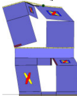
Analisi "Pushover -Y Acc - e". Configurazione della parete 13 in corrispondenza della capacità relativa allo stato limite SLV (passo 204).
