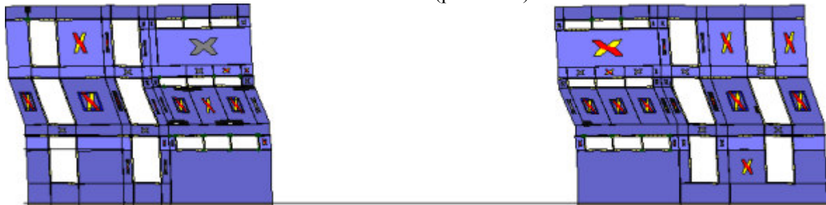
Analisi "Pushover -X Acc - e". Configurazione della parete 26 in corrispondenza della capacità relativa allo stato limite SLV (passo 134).
