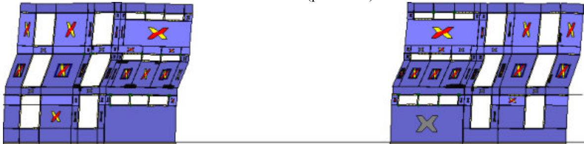
Analisi "Pushover +X Acc". Configurazione della parete 26 in corrispondenza della capacità relativa allo stato limite SLV (passo 328).
