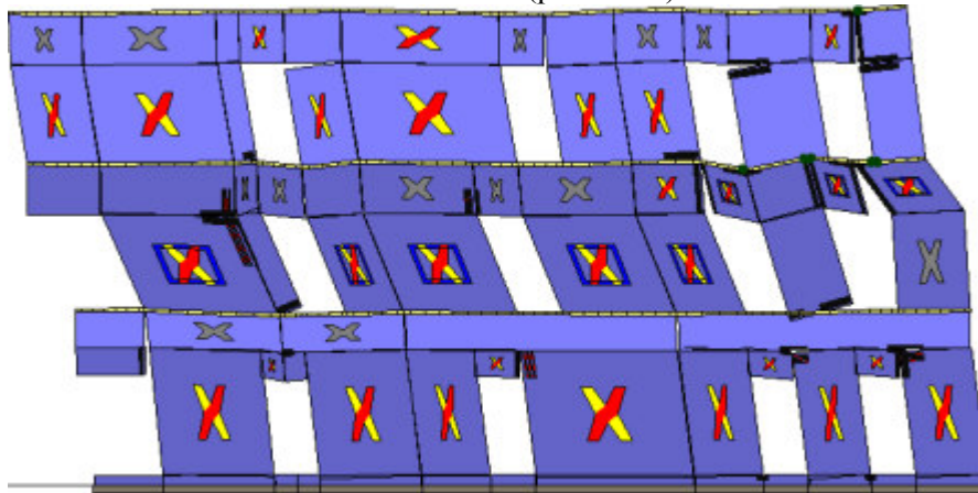
Analisi "Pushover -Y Acc". Configurazione della parete 18 in corrispondenza della capacità relativa allo stato limite SLV (passo 125).
