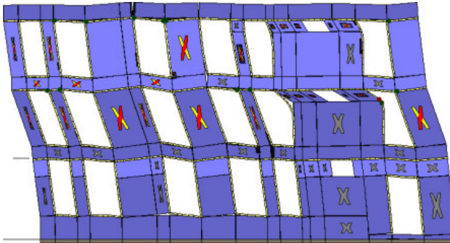
Analisi "Pushover -Y Acc - e". Configurazione della parete 31 in corrispondenza della capacità relativa allo stato limite SLV (passo 204).
