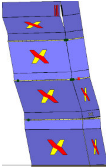
Analisi "Pushover +Y Acc + e". Configurazione della parete 2 in corrispondenza della capacità relativa allo stato limite SLV (passo 255).
