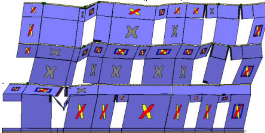
Analisi "Pushover +Y Acc". Configurazione della parete 18 in corrispondenza della capacità relativa allo stato limite SLV (passo 228).
