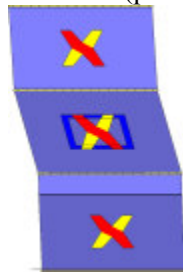
Analisi "Pushover -X Acc + e". Configurazione della parete 35 in corrispondenza della capacità relativa allo stato limite SLV (passo 135).
