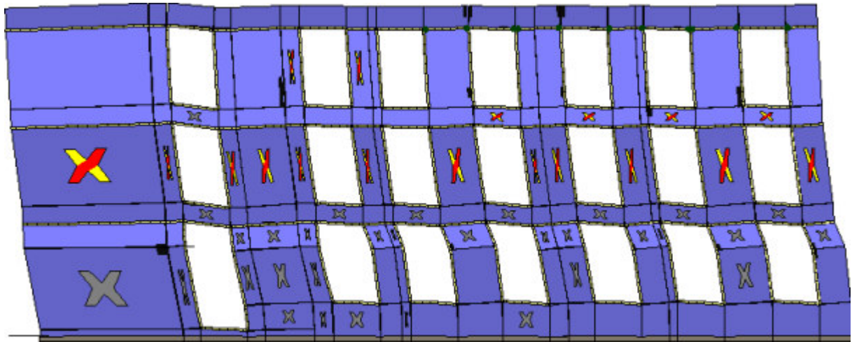
Analisi "Pushover -Y Massa + e". Configurazione della parete 34 in corrispondenza della capacità relativa allo stato limite SLV (passo 80).
