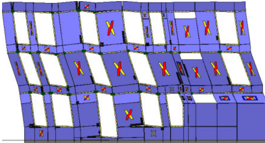
Analisi "Pushover -Y Acc". Configurazione della parete 22 in corrispondenza della capacità relativa allo stato limite SLV (passo 125).
