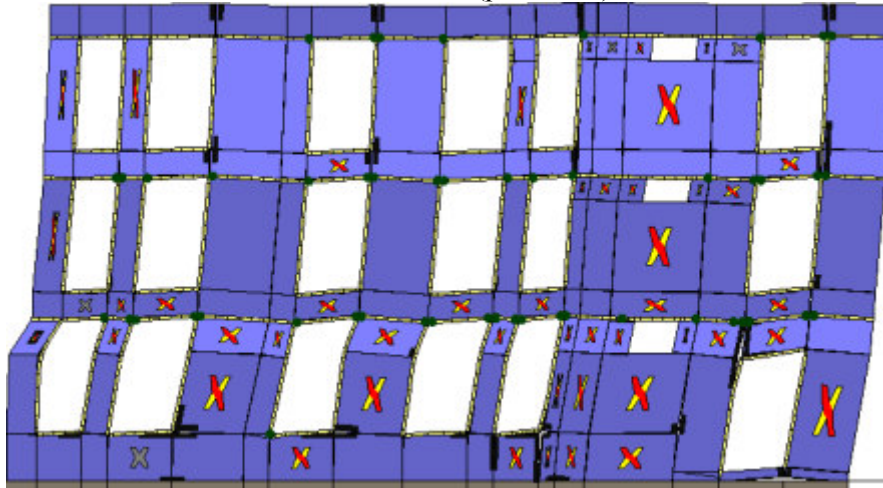
Analisi "Pushover +Y Massa". Configurazione della parete 31 in corrispondenza della capacità relativa allo stato limite SLV (passo 203).
