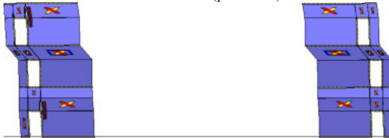
Analisi "Pushover -X Acc + e". Configurazione della parete 25 in corrispondenza della capacità relativa allo stato limite SLV (passo 135).
