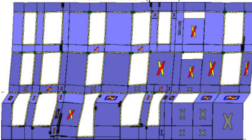
Analisi "Pushover +Y Massa + e". Configurazione della parete 22 in corrispondenza della capacità relativa allo stato limite SLV (passo 72).
