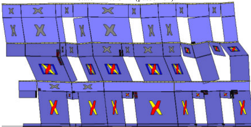
Analisi "Pushover -Y Acc - e". Configurazione della parete 18 in corrispondenza della capacità relativa allo stato limite SLV (passo 204).
