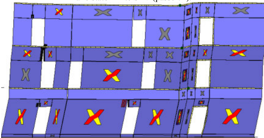
Analisi "Pushover +Y Massa + e". Configurazione della parete 21 in corrispondenza della capacità relativa allo stato limite SLV (passo 72).
