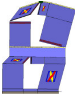
Analisi "Pushover +Y Acc + e". Configurazione della parete 13 in corrispondenza della capacità relativa allo stato limite SLV (passo 255).
