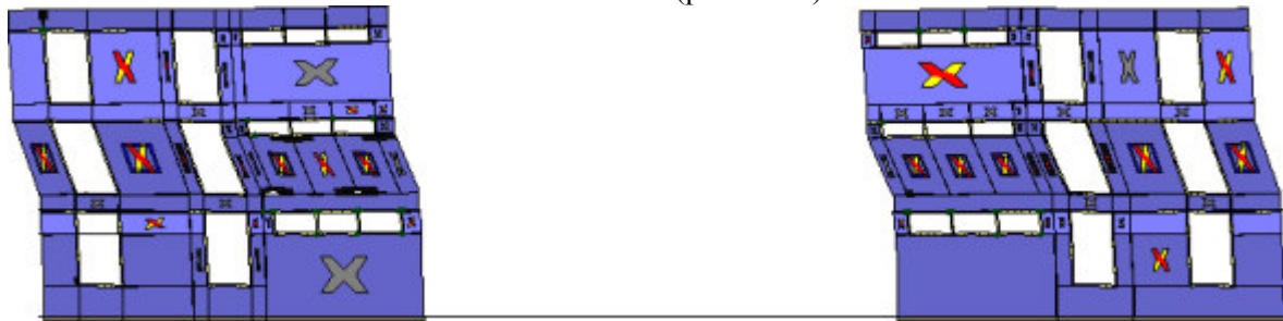
Analisi "Pushover -X Acc". Configurazione della parete 26 in corrispondenza della capacità relativa allo stato limite SLV (passo 299).
