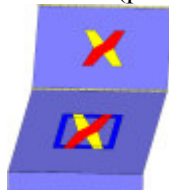
Analisi "Pushover +X Acc". Configurazione della parete 8 in corrispondenza della capacità relativa allo stato limite SLV (passo 328).
