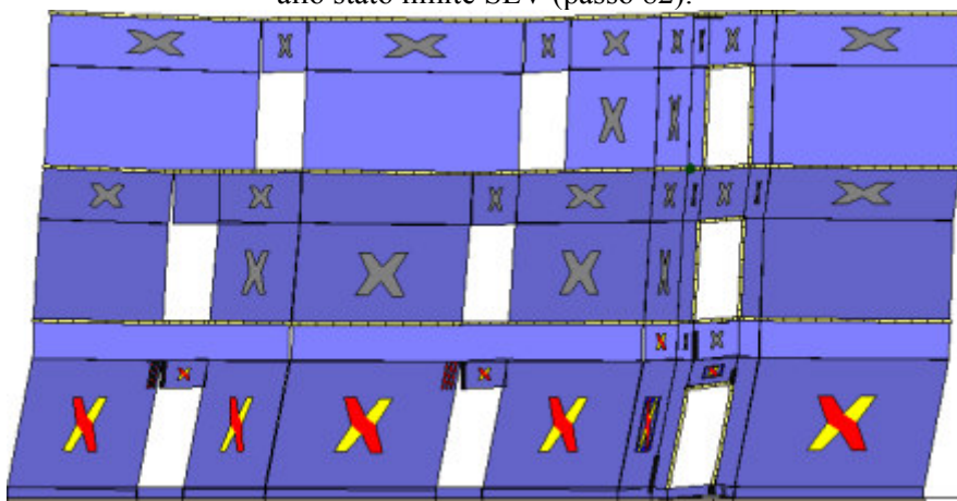
Analisi "Pushover +Y Massa - e". Configurazione della parete 32 in corrispondenza della capacità relativa allo stato limite SLV (passo 82).
