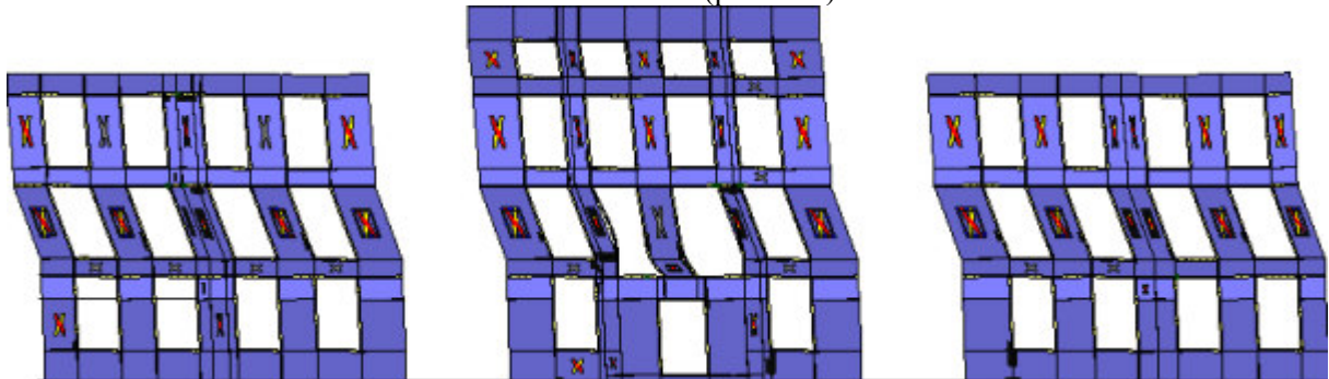
Analisi "Pushover +X Acc + e". Configurazione della parete 8 in corrispondenza della capacità relativa allo stato limite SLV (passo 86).
