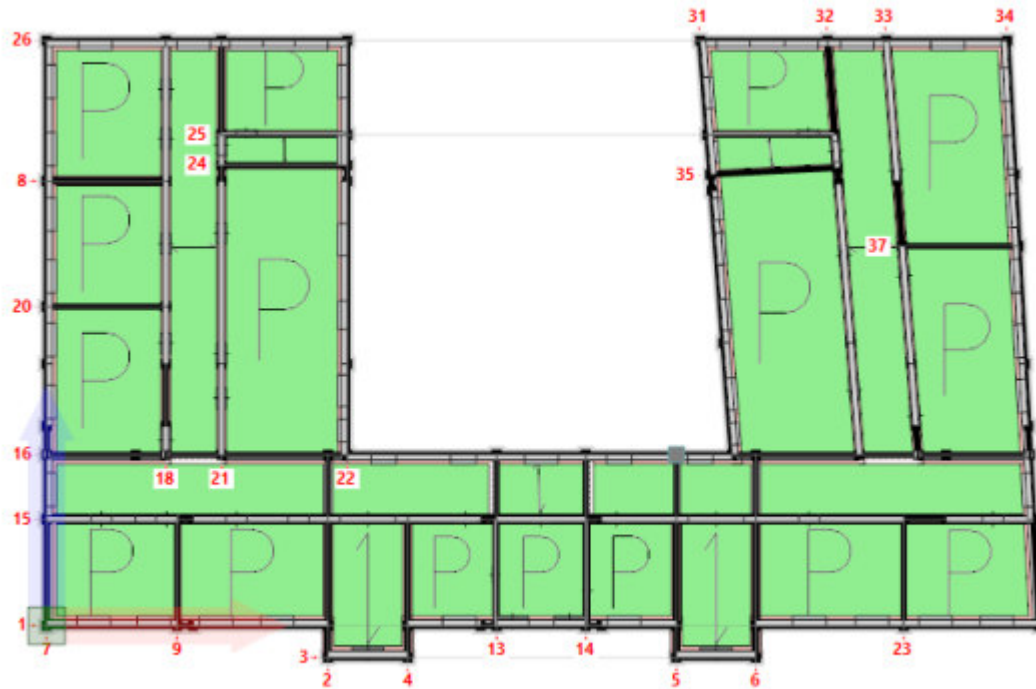
Pianta a quota 1040 cm con l'indicazione dei numeri attribuiti alle pareti.
