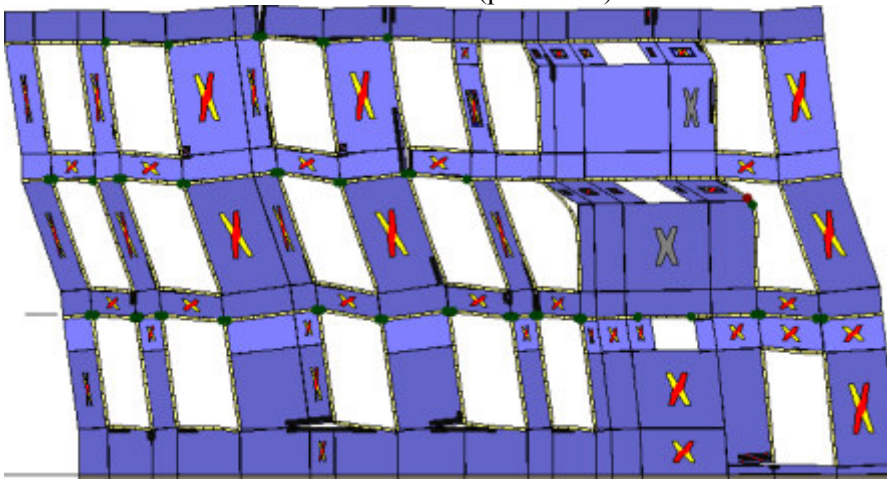
Analisi "Pushover -Y Acc". Configurazione della parete 31 in corrispondenza della capacità relativa allo stato limite SLV (passo 125).
