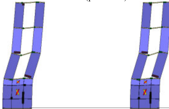
Analisi "Pushover +X Acc". Configurazione della parete 3 in corrispondenza della capacità relativa allo stato limite SLV (passo 328).
