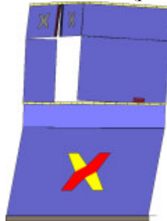
Analisi "Pushover +Y Massa - e". Configurazione della parete 14 in corrispondenza della capacità relativa allo stato limite SLV (passo 82).
