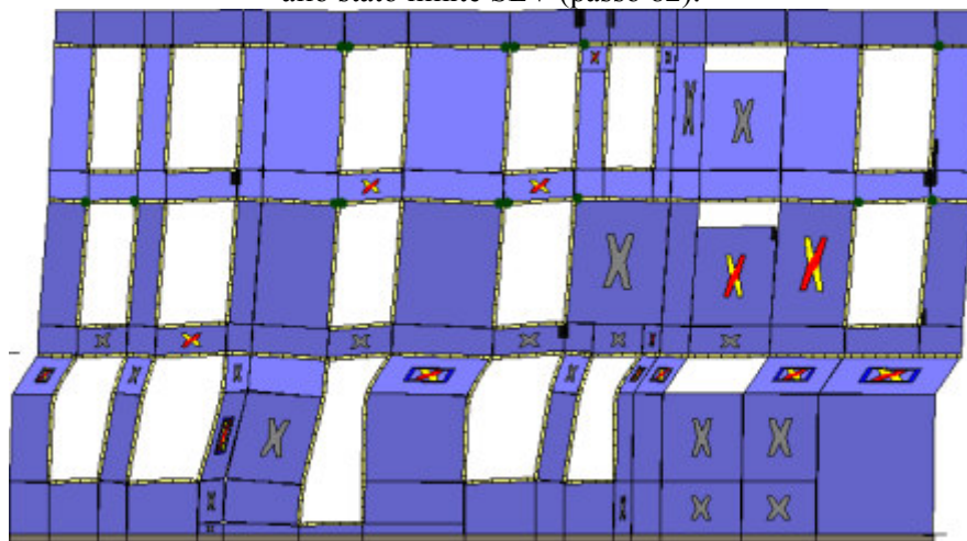
Analisi "Pushover +Y Massa - e". Configurazione della parete 22 in corrispondenza della capacità relativa allo stato limite SLV (passo 82).
