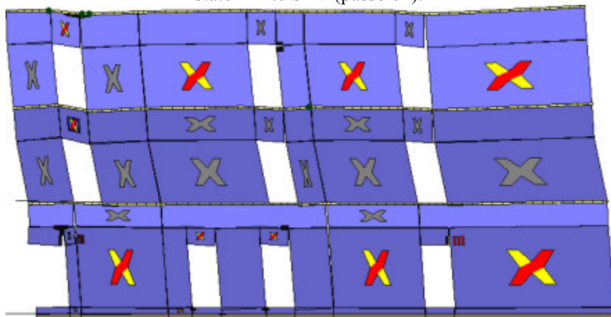
Analisi "Pushover -Y Acc + e". Configurazione della parete 33 in corrispondenza della capacità relativa allo stato limite SLV (passo 64).
