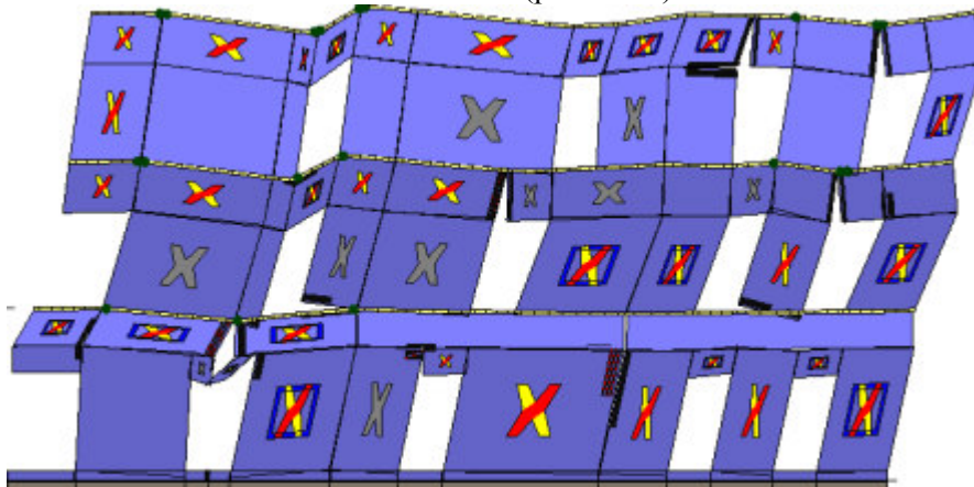
Analisi "Pushover +Y Acc + e". Configurazione della parete 18 in corrispondenza della capacità relativa allo stato limite SLV (passo 255).
