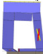
Analisi "Pushover -Y Acc + e". Configurazione della parete 29 in corrispondenza della capacità relativa allo stato limite SLV (passo 64).
