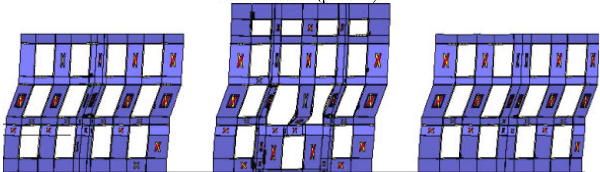
Analisi "Pushover +X Massa - e". Configurazione della parete 1 in corrispondenza della capacità relativa allo stato limite SLV (passo 84).
