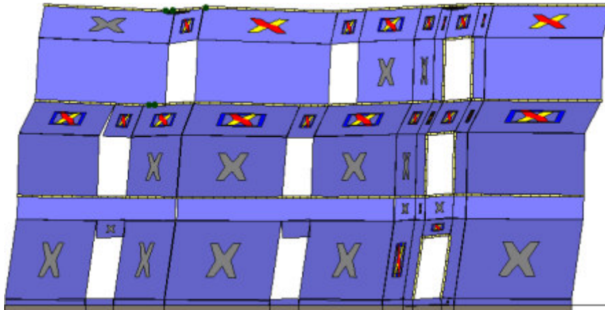
Analisi "Pushover +Y Acc - e". Configurazione della parete 32 in corrispondenza della capacità relativa allo stato limite SLV (passo 157).
