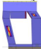
Analisi "Pushover +Y Acc - e". Configurazione della parete 30 in corrispondenza della capacità relativa allo stato limite SLV (passo 157).
