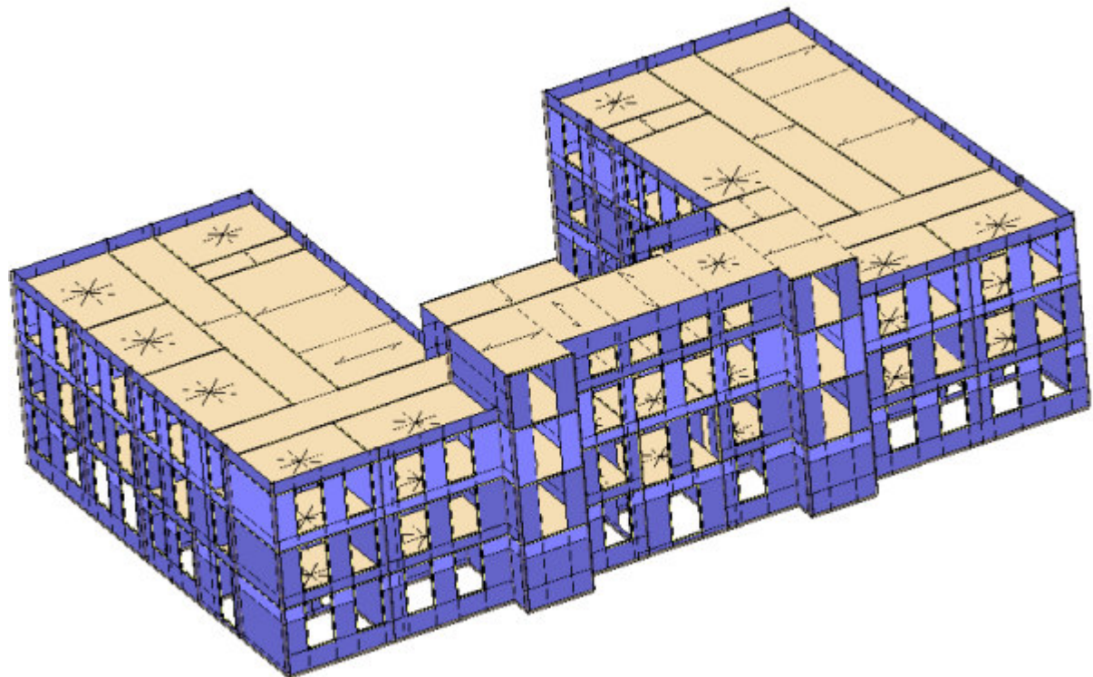
Modello 3DMacro - Vista assometrica 2.
