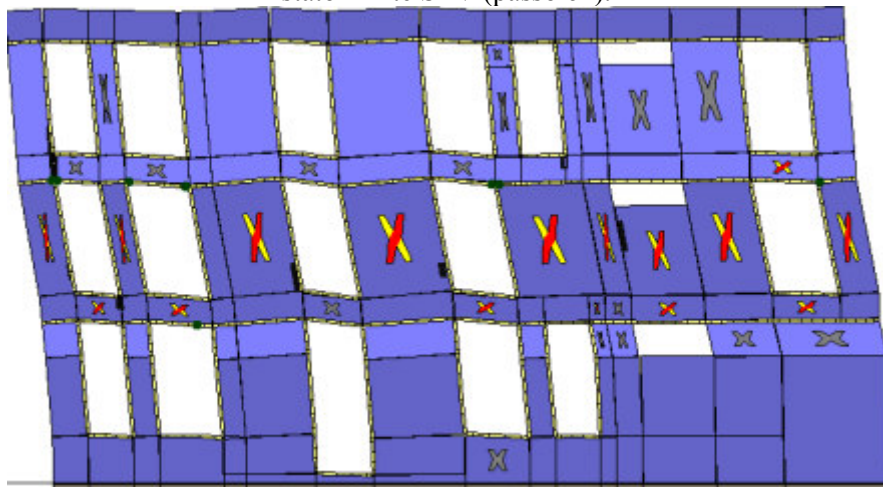
Analisi "Pushover -Y Acc + e". Configurazione della parete 22 in corrispondenza della capacità relativa allo stato limite SLV (passo 64).
