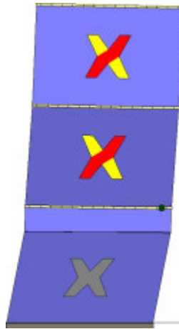
Analisi "Pushover +Y Massa - e". Configurazione della parete 9 in corrispondenza della capacità relativa allo stato limite SLV (passo 82).
