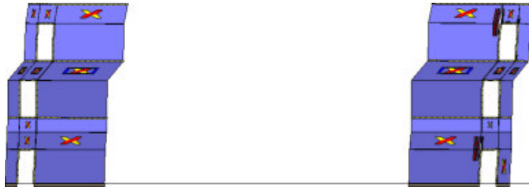
Analisi "Pushover +X Acc + e". Configurazione della parete 25 in corrispondenza della capacità relativa allo stato limite SLV (passo 86).
