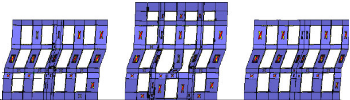
Analisi "Pushover +X Massa". Configurazione della parete 1 in corrispondenza della capacità relativa allo stato limite SLV (passo 84).
