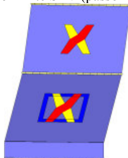
Analisi "Pushover +Y Acc". Configurazione della parete 23 in corrispondenza della capacità relativa allo stato limite SLV (passo 228).
