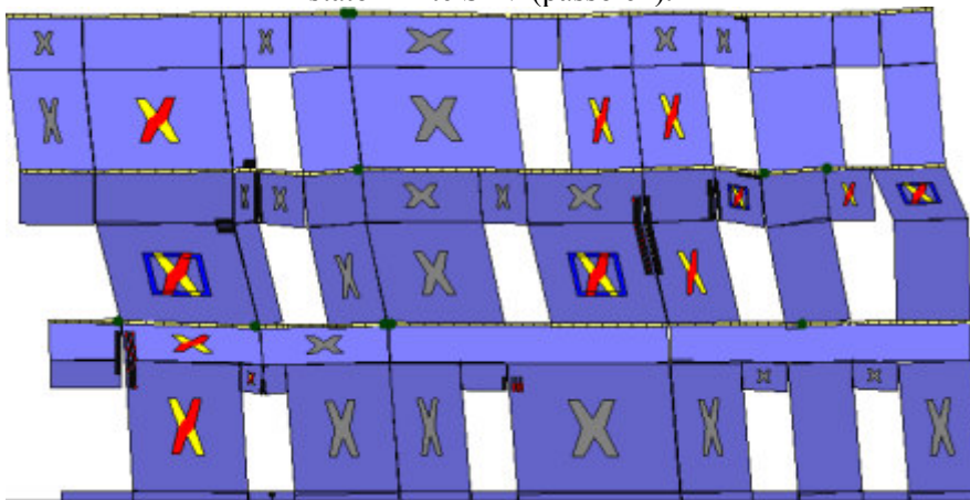
Analisi "Pushover -Y Acc + e". Configurazione della parete 18 in corrispondenza della capacità relativa allo stato limite SLV (passo 64).
