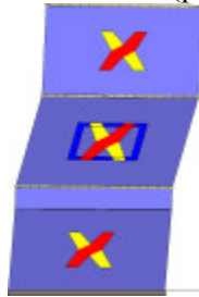
Analisi "Pushover +X Massa - e". Configurazione della parete 35 in corrispondenza della capacità relativa allo stato limite SLV (passo 84).
