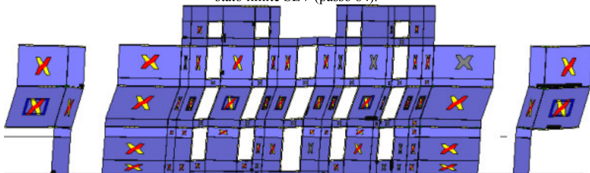
Analisi "Pushover +X Massa". Configurazione della parete 16 in corrispondenza della capacità relativa allo stato limite SLV (passo 84).
