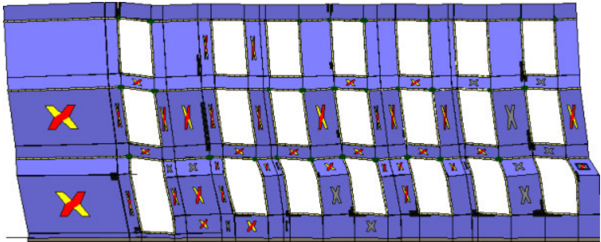
Analisi "Pushover -Y Massa". Configurazione della parete 34 in corrispondenza della capacità relativa allo stato limite SLV (passo 115).
