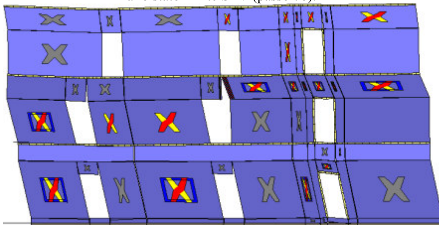
Analisi "Pushover -Y Massa - e". Configurazione della parete 32 in corrispondenza della capacità relativa allo stato limite SLV (passo 78).
