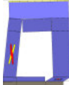
Analisi "Pushover -Y Acc + e". Configurazione della parete 30 in corrispondenza della capacità relativa allo stato limite SLV (passo 64).
