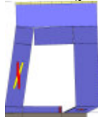
Analisi "Pushover -Y Acc - e". Configurazione della parete 30 in corrispondenza della capacità relativa allo stato limite SLV (passo 204).
