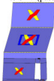
Analisi "Pushover +X Acc". Configurazione della parete 24 in corrispondenza della capacità relativa allo stato limite SLV (passo 328).
