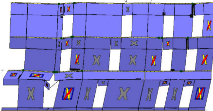
Analisi "Pushover +Y Massa - e". Configurazione della parete 18 in corrispondenza della capacità relativa allo stato limite SLV (passo 82).
