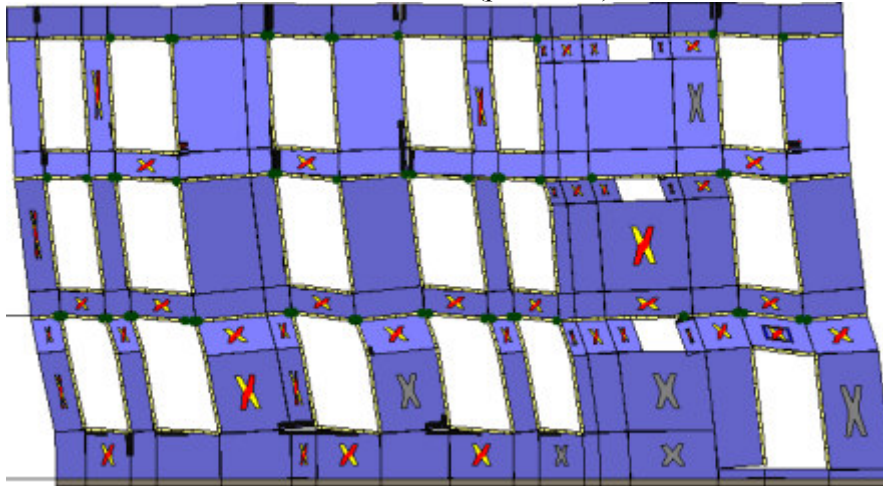
Analisi "Pushover -Y Massa". Configurazione della parete 31 in corrispondenza della capacità relativa allo stato limite SLV (passo 115).
