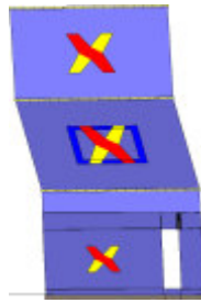
Analisi "Pushover -X Acc - e". Configurazione della parete 24 in corrispondenza della capacità relativa allo stato limite SLV (passo 134).
