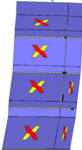
Analisi "Pushover -Y Massa". Configurazione della parete 2 in corrispondenza della capacità relativa allo stato limite SLV (passo 115).
