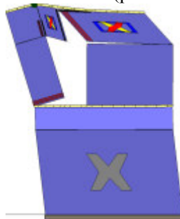
Analisi "Pushover -Y Acc - e". Configurazione della parete 14 in corrispondenza della capacità relativa allo stato limite SLV (passo 204).
