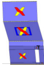
Analisi "Pushover -X Massa - e". Configurazione della parete 24 in corrispondenza della capacità relativa allo stato limite SLV (passo 79).
