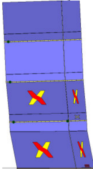
Analisi "Pushover +Y Massa + e". Configurazione della parete 5 in corrispondenza della capacità relativa allo stato limite SLV (passo 72).
