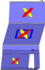
Analisi "Pushover +X Massa - e". Configurazione della parete 24 in corrispondenza della capacità relativa allo stato limite SLV (passo 84).
