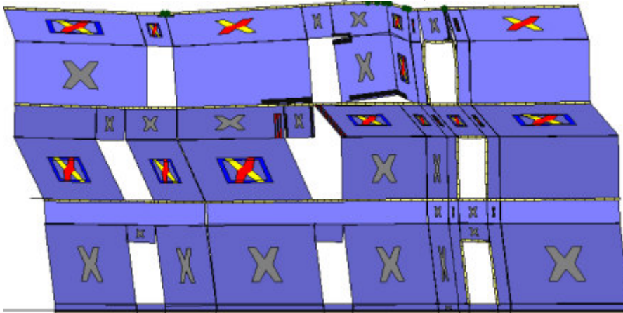
Analisi "Pushover -Y Acc - e". Configurazione della parete 32 in corrispondenza della capacità relativa allo stato limite SLV (passo 204).
