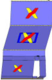
Analisi "Pushover +X Massa + e". Configurazione della parete 24 in corrispondenza della capacità relativa allo stato limite SLV (passo 83).
