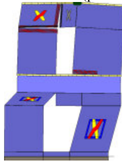
Analisi "Pushover +Y Massa - e". Configurazione della parete 13 in corrispondenza della capacità relativa allo stato limite SLV (passo 82).
