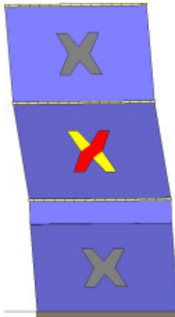
Analisi "Pushover -Y Acc + e". Configurazione della parete 9 in corrispondenza della capacità relativa allo stato limite SLV (passo 64).
