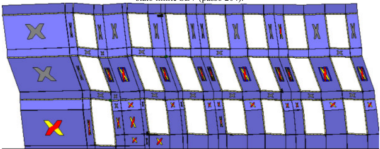
Analisi "Pushover -Y Acc - e". Configurazione della parete 7 in corrispondenza della capacità relativa allo stato limite SLV (passo 204).
