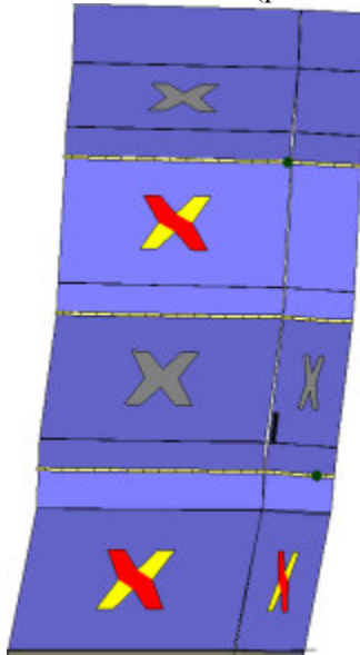
Analisi "Pushover -Y Massa + e". Configurazione della parete 2 in corrispondenza della capacità relativa allo stato limite SLV (passo 80).
