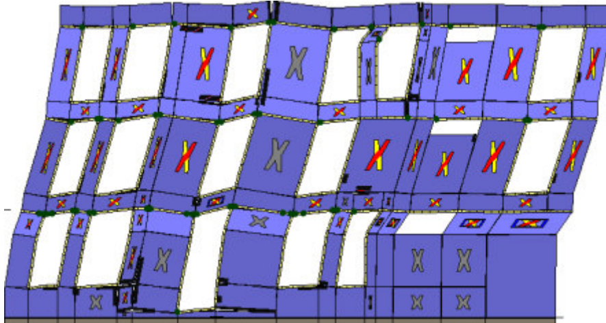
Analisi "Pushover +Y Acc + e". Configurazione della parete 22 in corrispondenza della capacità relativa allo stato limite SLV (passo 255).
