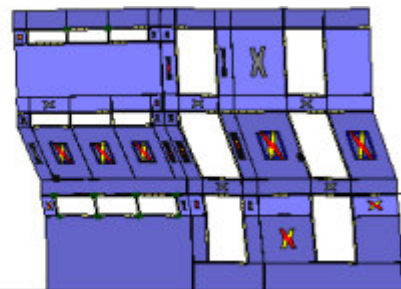
Analisi "Pushover -X Massa". Configurazione della parete 25 in corrispondenza della capacità relativa allo stato limite SLV (passo 79).
