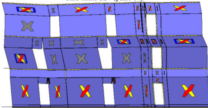
Analisi "Pushover -Y Acc + e". Configurazione della parete 32 in corrispondenza della capacità relativa allo stato limite SLV (passo 64).
