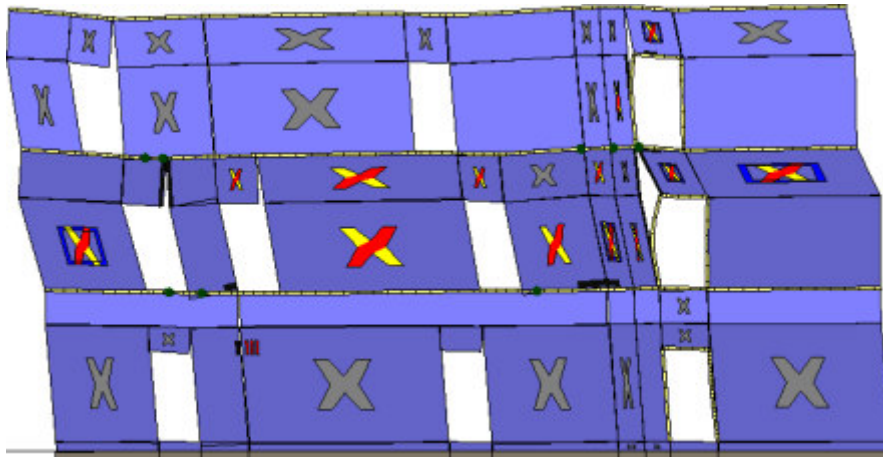
Analisi "Pushover -Y Acc + e". Configurazione della parete 21 in corrispondenza della capacità relativa allo stato limite SLV (passo 64).
