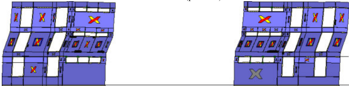
Analisi "Pushover +X Acc + e". Configurazione della parete 26 in corrispondenza della capacità relativa allo stato limite SLV (passo 86).
