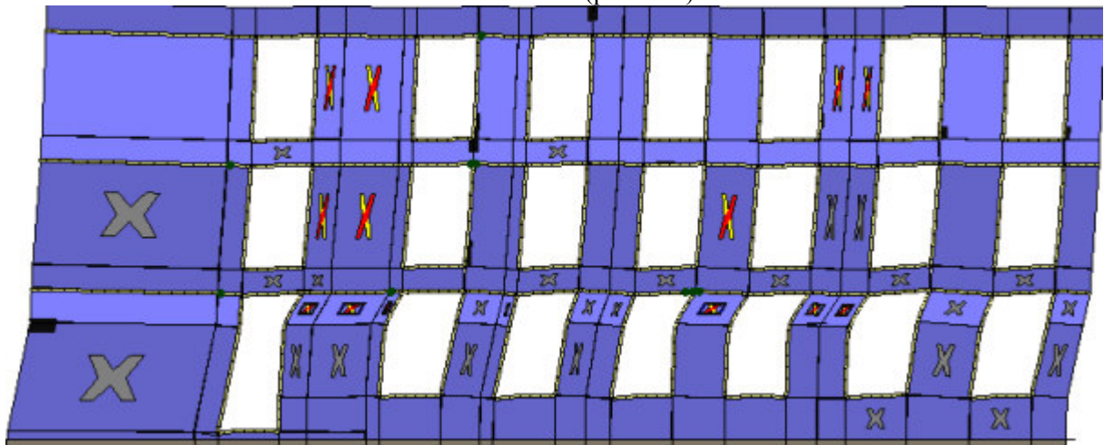
Analisi "Pushover +Y Massa - e". Configurazione della parete 7 in corrispondenza della capacità relativa allo stato limite SLV (passo 82).
