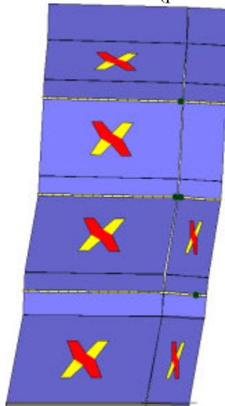
Analisi "Pushover -Y Massa - e". Configurazione della parete 2 in corrispondenza della capacità relativa allo stato limite SLV (passo 78).
