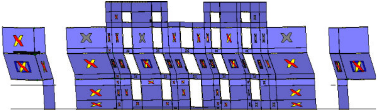
Analisi "Pushover -X Massa". Configurazione della parete 16 in corrispondenza della capacità relativa allo stato limite SLV (passo 79).
