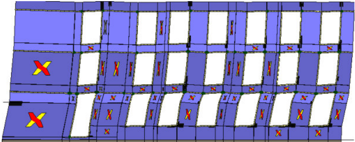
Analisi "Pushover +Y Massa + e". Configurazione della parete 34 in corrispondenza della capacità relativa allo stato limite SLV (passo 72).
