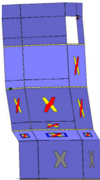
Analisi "Pushover -Y Massa - e". Configurazione della parete 4 in corrispondenza della capacità relativa allo stato limite SLV (passo 78).
