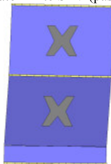
Analisi "Pushover +Y Massa - e". Configurazione della parete 23 in corrispondenza della capacità relativa allo stato limite SLV (passo 82).
