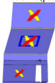
Analisi "Pushover +X Acc - e". Configurazione della parete 24 in corrispondenza della capacità relativa allo stato limite SLV (passo 86).
