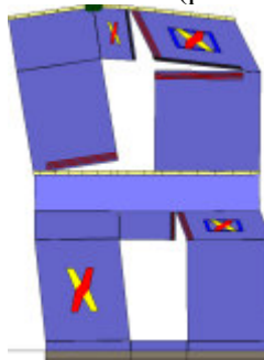
Analisi "Pushover -Y Acc + e". Configurazione della parete 13 in corrispondenza della capacità relativa allo stato limite SLV (passo 64).
