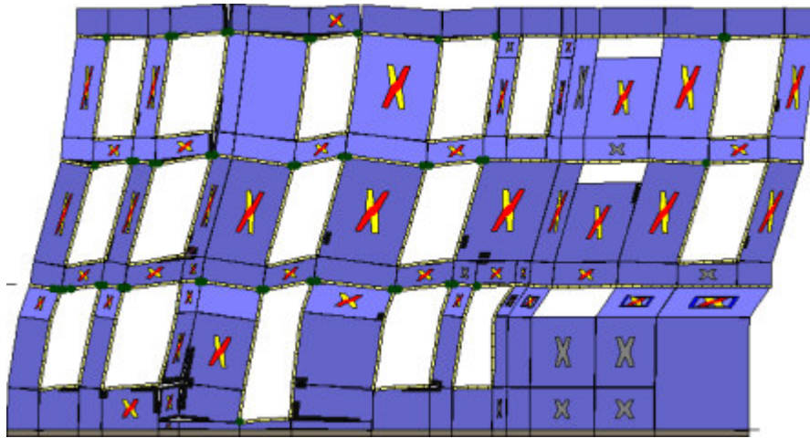
Analisi "Pushover +Y Acc". Configurazione della parete 22 in corrispondenza della capacità relativa allo stato limite SLV (passo 228).
