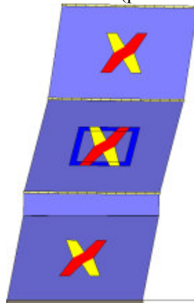
Analisi "Pushover +Y Acc + e". Configurazione della parete 9 in corrispondenza della capacità relativa allo stato limite SLV (passo 255).
