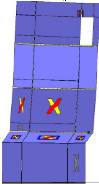
Analisi "Pushover +Y Massa - e". Configurazione della parete 4 in corrispondenza della capacità relativa allo stato limite SLV (passo 82).
