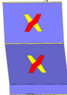
Analisi "Pushover -Y Massa". Configurazione della parete 23 in corrispondenza della capacità relativa allo stato limite SLV (passo 115).
