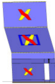
Analisi "Pushover -X Acc". Configurazione della parete 24 in corrispondenza della capacità relativa allo stato limite SLV (passo 299).
