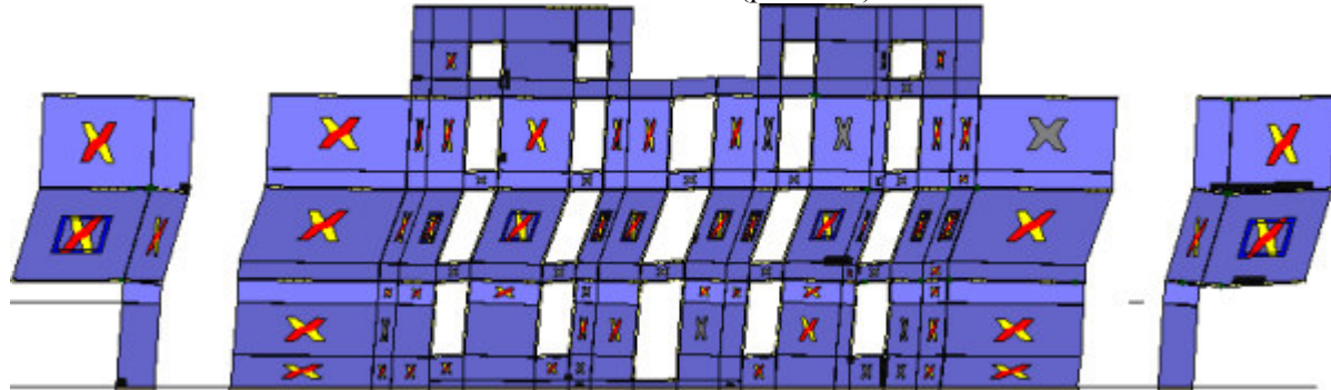
Analisi "Pushover +X Massa - e". Configurazione della parete 16 in corrispondenza della capacità relativa allo stato limite SLV (passo 84).
