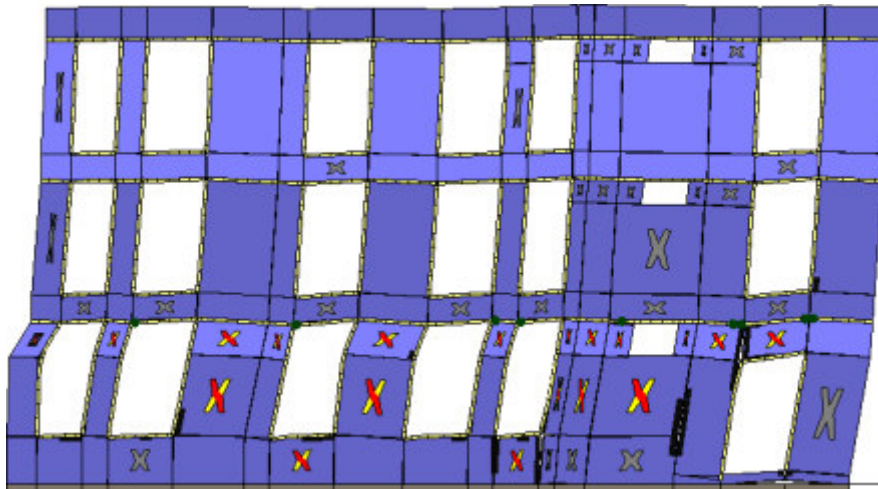
Analisi "Pushover +Y Massa - e". Configurazione della parete 31 in corrispondenza della capacità relativa allo stato limite SLV (passo 82).
