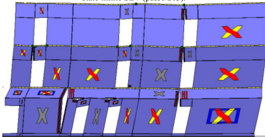
Analisi "Pushover +Y Massa". Configurazione della parete 33 in corrispondenza della capacità relativa allo stato limite SLV (passo 203).
