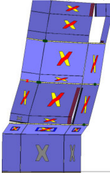
Analisi "Pushover +Y Acc + e". Configurazione della parete 4 in corrispondenza della capacità relativa allo stato limite SLV (passo 255).
